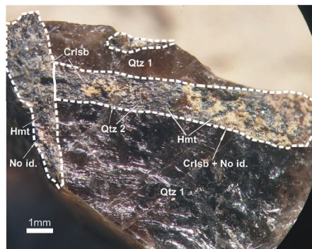
Figura 7. Fotomicrografía de cristales prismáticos tabulares de mineral no identificado (¿grupo de la columbita?) reemplazado pseudomórficamente por agregados de hematita especular (Hmt) + cuarzo (Qtz 2) + carlosbarbosaíta (CrIsb) + mineral no identificado de aspecto arcilloso (No id.). El mineral reemplazado se halla incluido en cuarzo ahumado (Qtz 1) en la zona externa del núcleo de cuarzo, hacia la zona feldespática y el granito porfírico encajonante.
