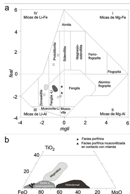
Figura 3. a) Valores microanalíticos (WDS) y campos composicionales de micas del plutón La Chinchilla registrados en el diagrama de micas dioctaédricas y trioctaédricas de Tischendorf (1997), mgli = (Mg+Li) y feal = (Fe+Ti+Mn+Al^{IV}) . Estrellas rellenas: facies porfírica de grano grueso (WP195), estrellas vacías: granito porfírico muscovitizado en borde externo de miarola, trinchera T4, WP160 (Bardelli 2014); área gris oscuro: facies equigranular miarolítica (Lira et al. 2015); área y cuadrados gris claro: facies no especificadas (Grosse et al. 2006; Grosse 2007); b) Relaciones Ti-Fe-Mg de las micas analizadas del plutón La Chinchilla en el esquema genético discriminador de Speer (1984).
