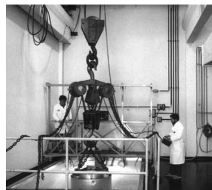
Contenedor blindado para transporte de ^{60}\text{Co} .
