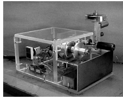
Proyecto Molibdeno 99 Máquina para corte y muestreo de régulos.
