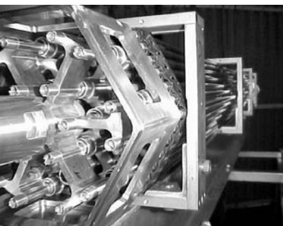
Prototipo del elemento combustible CAREM
