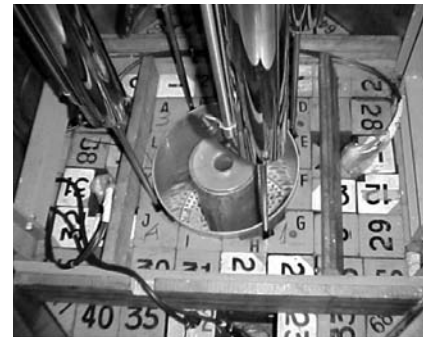
Núcleo del Reactor de Investigación RA-0 Universidad Nacional de Córdoba
