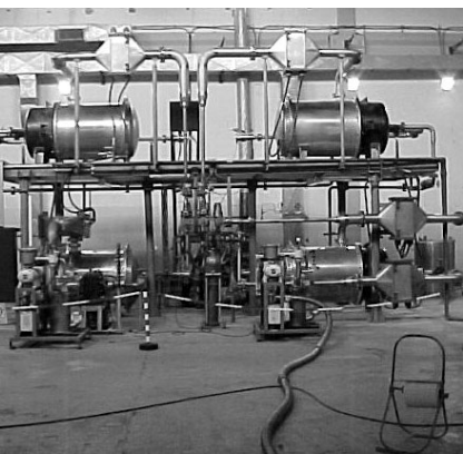
Imagen del "mock-up" SIGMA, en funcionamiento. Complejo Tecnológico Pilcaniyeu.
