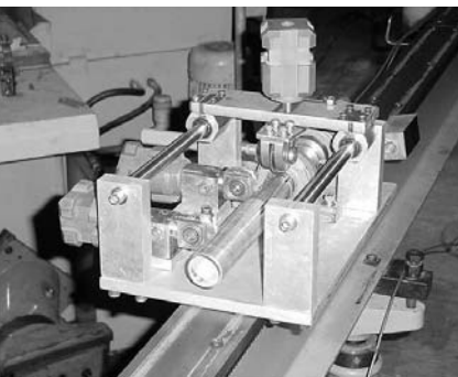
Proyecto Molibdeno 99. Máquina para corte de blancos postirradiación.
