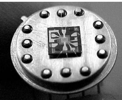
Sensor encapsulado con el conexión de hilos de oro de 50 mm.
