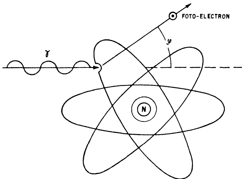
Fig. 4.12 Esquema del efecto fotoeléctrico.
