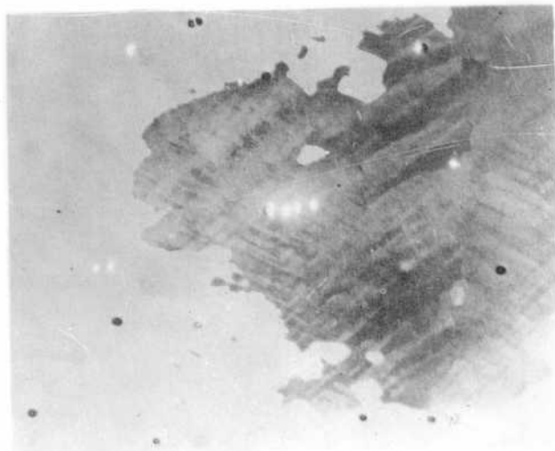
b) Même plage que la figure 6(a) après un nouveau recuit de 15' à 400°C. Lumière polarisée.
