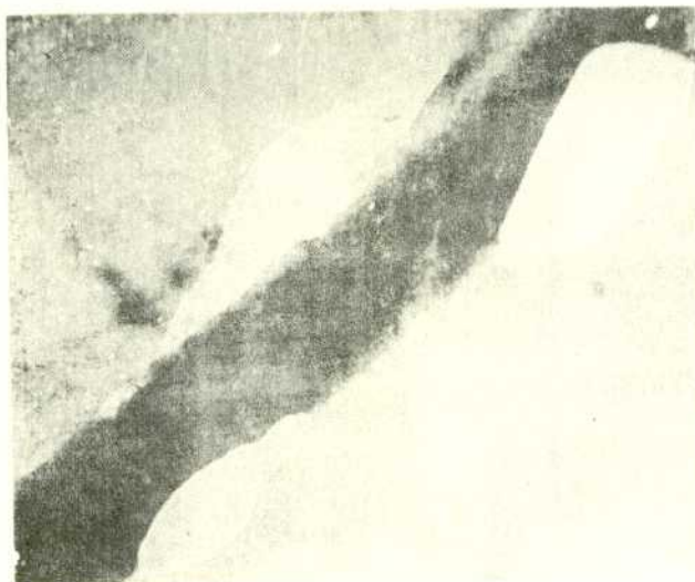
Figure 16.- Monocrystal déformé par traction 55%. Recuit 16 h à 300°C. Germination aux sous-joints des bandes de pliage compensé. Lumière polarisée.
