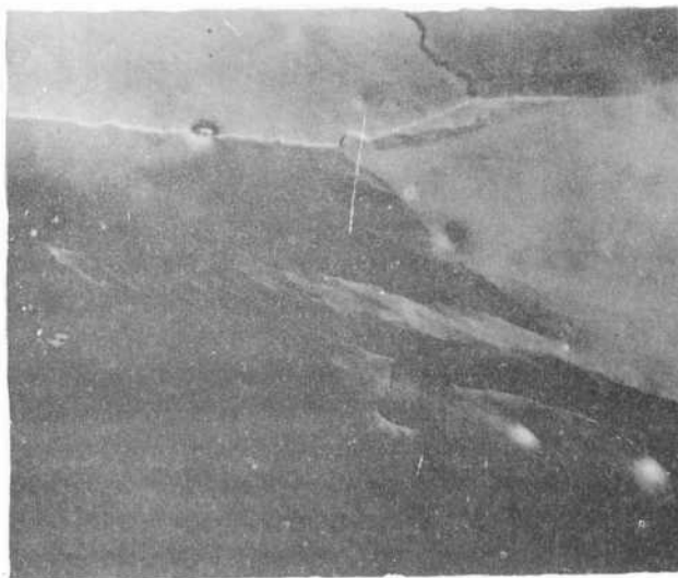
Figure 5.- Aluminium déformé 30% par impact recuit 1 h à 300°C. Migration des sous-joints CFIN G = 330
