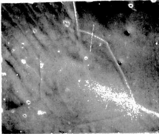
Figure 10.- Al déformé par laminage 30%. Recuit 1 h à 300°C. Germination dans un point triple. CFIN G= 700
