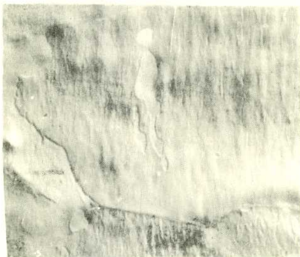
Figure 14.- Al déformé par laminage 30%. Recuit 1 h à 300°C. Germination à l'intérieur du grain. CFIN
