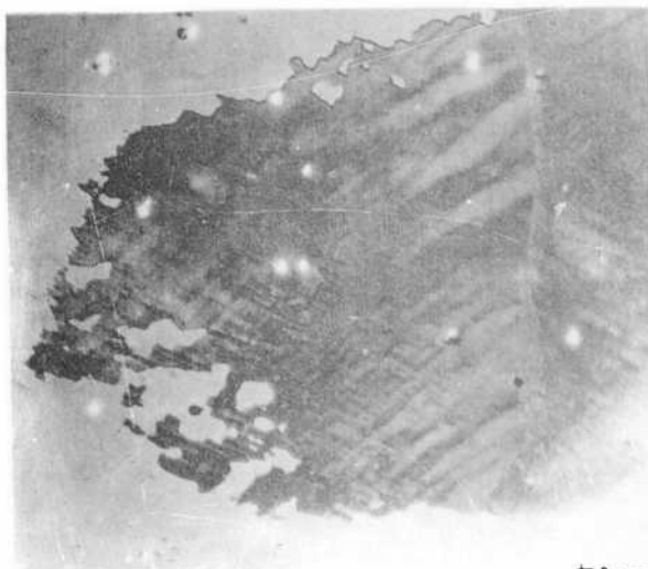
a) Aluminium déformé par traction 30% et recuit \frac{1}{2} h à 300°C. Croissance induite des grains. Lumière polarisée.
