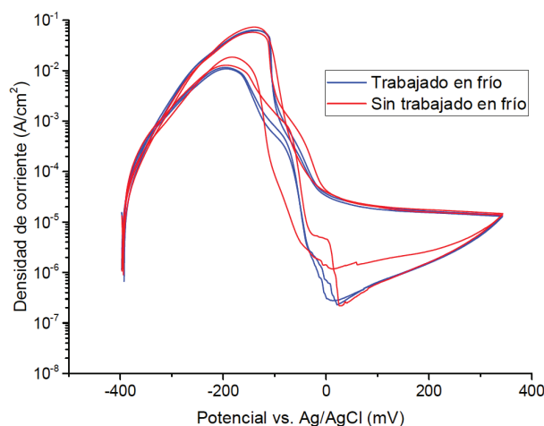
Figura 15. Curvas de DL-EPR en probetas sensibilizadas durante 2 horas a 677 °C para evaluar el efecto del trabajado en frío.
