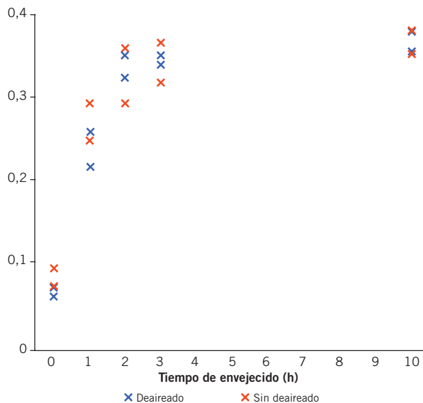
Figura 13. Resultados de DOS obtenidos a partir de mediciones de DL-EPR para evaluar el efecto del deaerado y del contenido de inclusiones.
