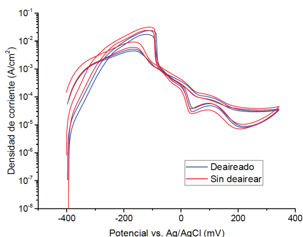
Figura 9. Curvas de DL-EPR en probetas sensibilizadas durante 1 hora a 677 °C para evaluar el efecto del deaireado y del contenido de inclusiones.
