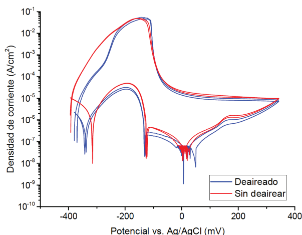
Figura 3. Curvas de DL-EPR en probetas solubilizadas para evaluar el efecto del deaireado.
