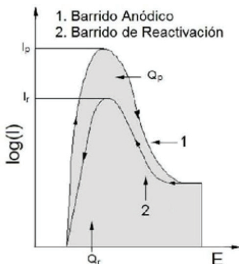
Figura 2. Curva esquemática del método DL-EPR (ISO 12732).
