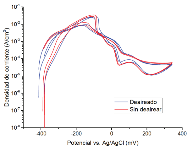
Figura 11. Curvas de DL-EPR en probetas sensibilizadas durante 3 horas a 677 °C para evaluar el efecto del deaerado y del contenido de inclusiones.
