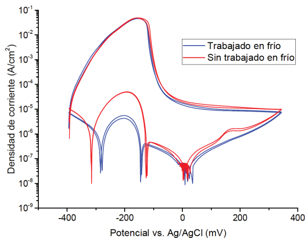
Figura 14. Curvas de DL-EPR en probetas solubilizadas para evaluar el efecto del trabajado en frío.
