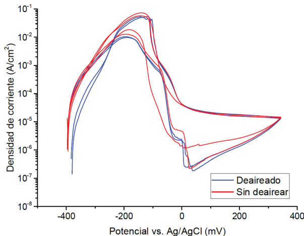
Figura 4. Curvas de DL-EPR en probetas sensibilizadas para evaluar el efecto del deaireado.
