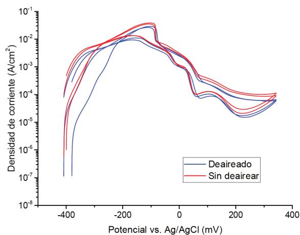
Figura 12. Curvas de DL-EPR en probetas sensibilizadas durante 10 horas a 677 °C para evaluar el efecto del deaerado y del contenido de inclusiones.
