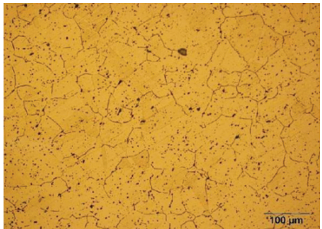
Figura 6. Microestructura del material con alto contenido de inclusiones. Corte transversal.
