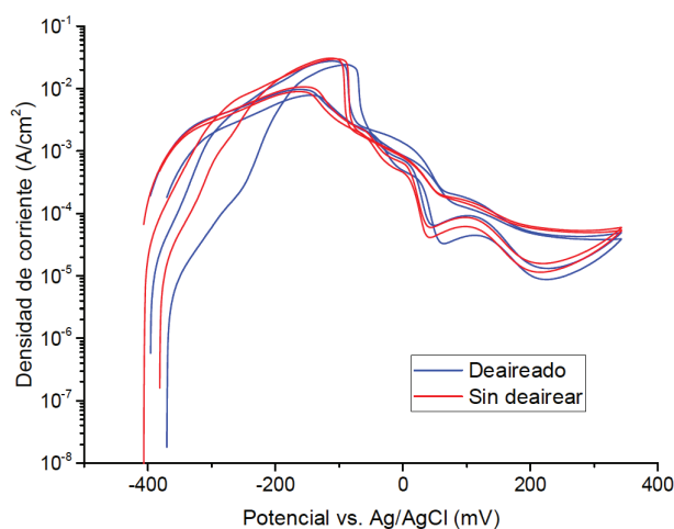
Figura 10. Curvas de DL-EPR en probetas sensibilizadas durante 2 horas a 677 °C para evaluar el efecto del deaireado y del contenido de inclusiones.
