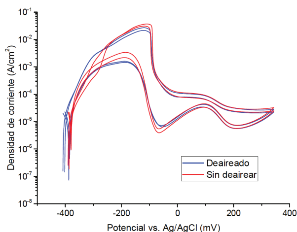
Figura 8. Curvas de DL-EPR en probetas solubilizadas para evaluar el efecto del deaireado y del contenido de inclusiones.
