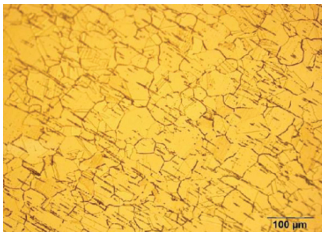
Figura 7. Microestructura del material con alto contenido de inclusiones. Corte longitudinal.
