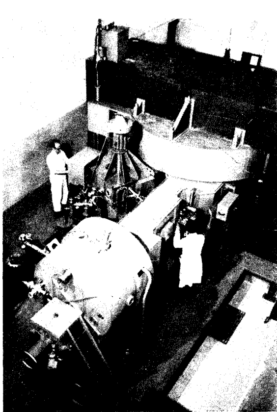
Enfoque del sincrociclotrón de Buenos Aires, de 30 MeV, mostrando el electroimán capaz de generar campos magnéticos de hasta 15 Kgauss.
