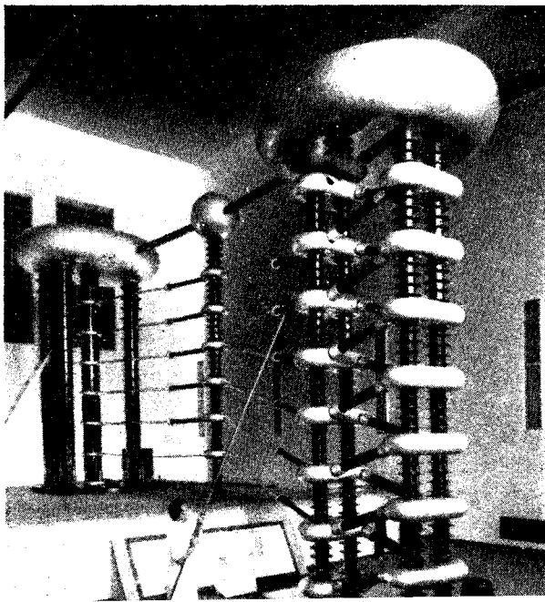
Accelerador Cockroft-Walton de 1,2 MeV existente en la sede central de la CNFA.
