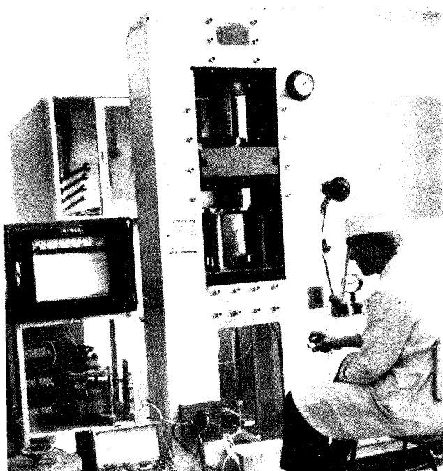
Presna de extrusión vertical utilizada en la fabricación de elementos combustibles para el RA-1.
