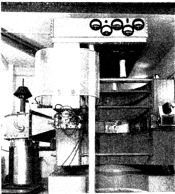
Separador electromagnético de isótopos (calutrón) construido en la CNEA.
