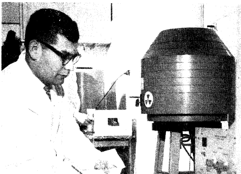
Equipo para medición de bajas actividades de emisores beta, utilizado para determinar el contenido de Estroncio-90, debido al fall-out, en muestras biológicas y demás medios antes mencionados.
