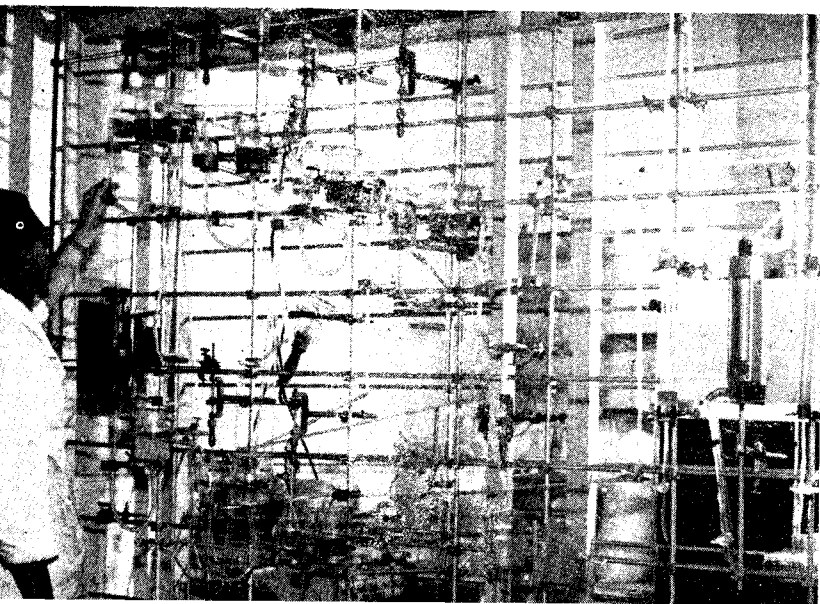
Equipo de ensayos hidrometalúrgicos para la extracción selectiva del uranio (escala de laboratorio).
