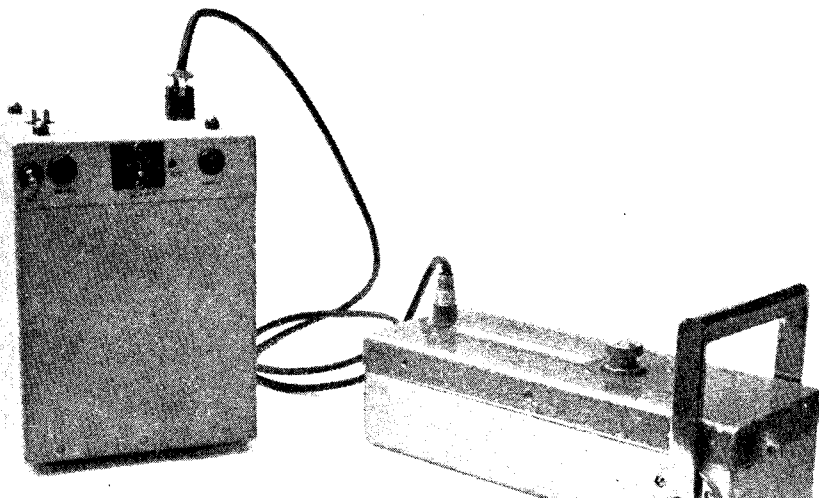
Medidor de suelos por reflexión radiactiva. Sonda y unidad de lectura del prototipo desarrollado y construido en la CNEA.
