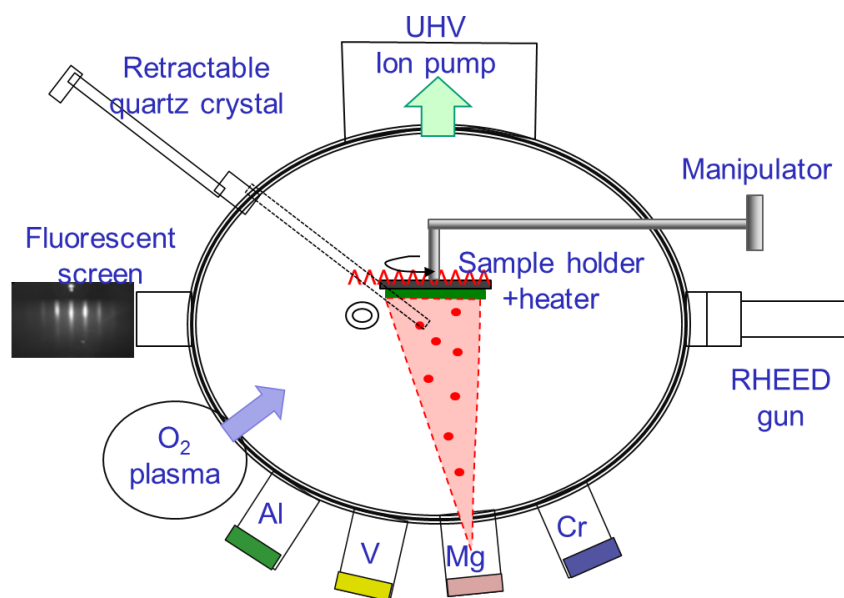
Figura A.5: Cámara de deposición por Molecular Beam Epitaxy . En el esquema se incluye el sistema de control de calidad de películas ( RHEED ). Gentileza de Mariela Menghini.
