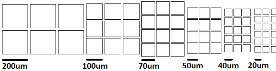
Figura 6.2: Litografía de los electrodos superiores para todas las muestras detalladas en la Tabla 6.1.
