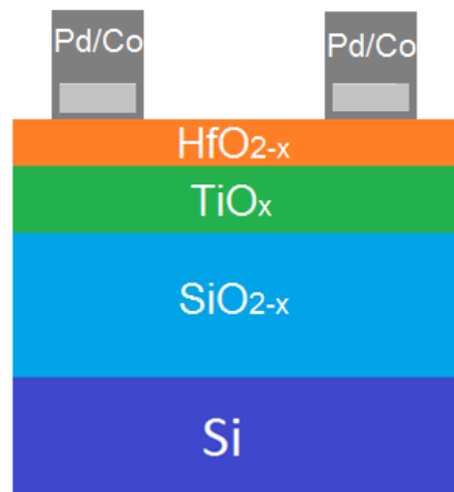
Figura 7.19: Apilamiento resultante del proceso de fabricación descrito en la Sección 7.2 en vistas de la caracterización estructural expuesta (Figs. 7.17 y 7.18).
