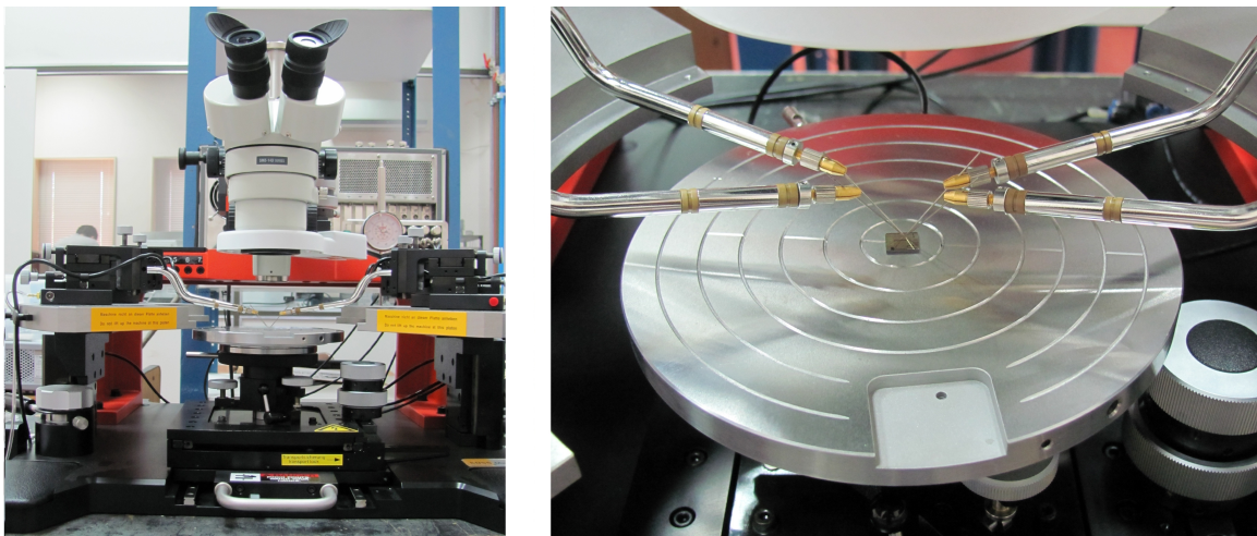
Figura 2.1: Fotografías de la estación de pruebas comercial ( Süss PM5 ) y detalle de las agujas microcontactoras, apoyadas sobre una muestra, sujetas a los manipuladores triaxiales.
