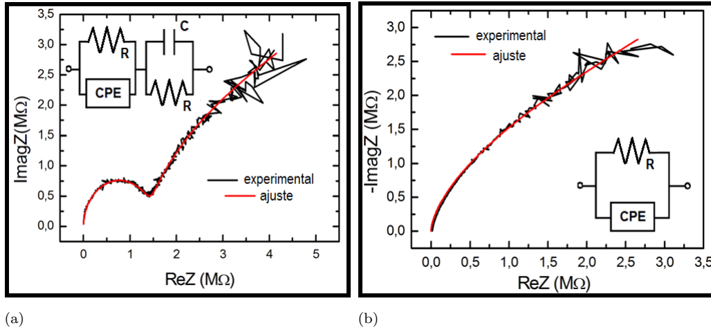
Figura 7.14: Cole-Cole para (a) HRS y (b) LRS . La figura se construye a partir de una medición de |Z| y \psi en función de la frecuencia con una condición de polarización y amplitud AC determinadas (en este caso: +4V y 5mV , respectivamente).
