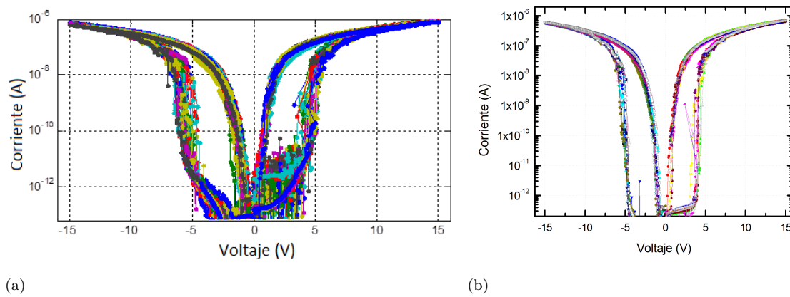
Figura 7.4: (a) Repetición de la medición I - V en un mismo dispositivo (20 ciclos). (b) Curva I - V registrada en dispositivos prístinos (20 dispositivos).
