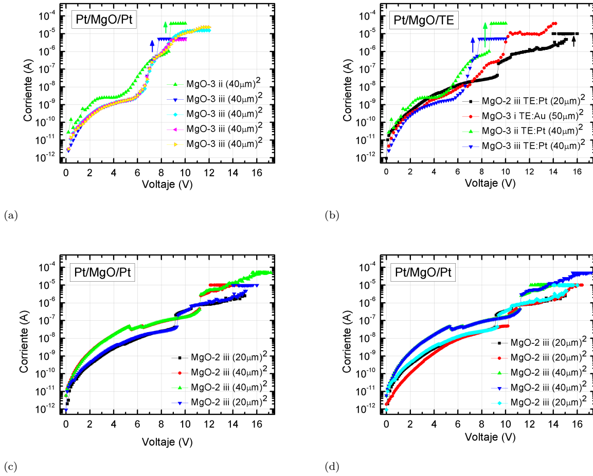
Figura 6.3: Corriente en función del voltaje para dispositivos prístinos. En cada subfigura se presentan dispositivos correspondientes a las características de deposición referidas en la Tabla 6.1. (a) Se analiza la incidencia de los cambios de presión de O_2 . También se aprecia que a condiciones idénticas, las curvas de distintos dispositivos se superponen. (b) Se comparan dispositivos con áreas y materiales de electrodo distintos. (c) Se representa el cambio debido al área del dispositivo. (d) Se comparan dispositivos fabricados con distintas condiciones de recocido. En todos los casos la señal se aplica en el electrodo superior mientras que el inferior permanece conectado a tierra.
