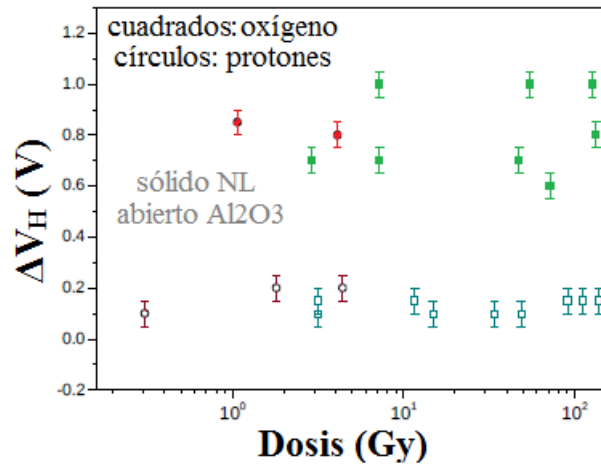
Figura 3.10: Evolución de la histéresis entre las curvas de IDA y VUELTA ( \Delta V_H ) en función de la dosis representada por los iones incidentes. Se presentan datos experimentales correspondientes a dos tipos de dieléctrico ( Al_2O_3 y NL ) y a las dos especies mencionadas analizadas: protones e iones oxígeno.
