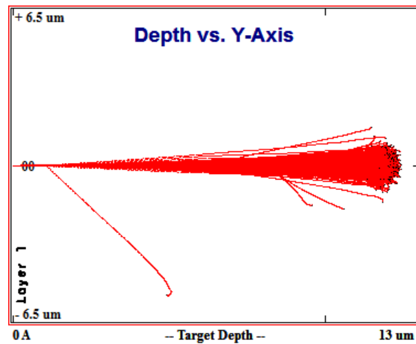
Figura 3.12: Simulación efectuada con el código SRIM de iones de oxígeno 20 MeV incidiendo sobre una película metálica de Al .
