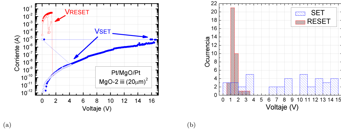
Figura 6.4: Operaciones de escritura ( SET ) y borrado ( RESET ) sucesivas, efectuadas en la muestra MgO-2 iii de la Tabla 6.1. En todos los casos el estímulo aplicado fue rampas de tensión, de manera que punto a punto se grafican los valores medidos de voltaje y corriente. El histograma incorporado refleja la dispersión entre las tensiones para las que se aprecian las distintas operaciones ( SET y RESET ). Comparativamente, la operación de escritura se presenta como un proceso más errático que la de borrado.
