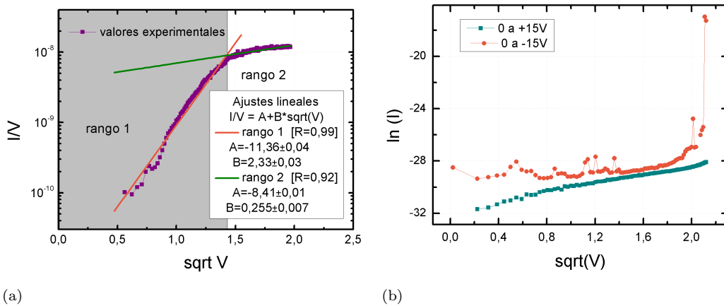
Figura 7.25: Dependencias típicas para analizar la pertinencia de los mecanismos: (a) Frenkel-Poole: \frac{I}{V} en función de \sqrt{V} y (b) Schottky: \ln(I) en función de \sqrt{V} . Al graficar de este modo se espera una dependencia lineal entre las abscisas y las ordenadas para cada caso.
