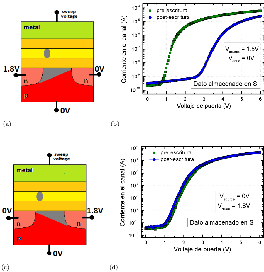
Figura 5.6: (a) Esquema del proceso de lectura en una condición particular del canal. (b) Lectura del dato guardado ( bit ). (c) Esquema del proceso de lectura en la condición del canal complementaria a la de la Fig. 5.6 (a). (d) Lectura del sitio complementario al que fue escrito.
