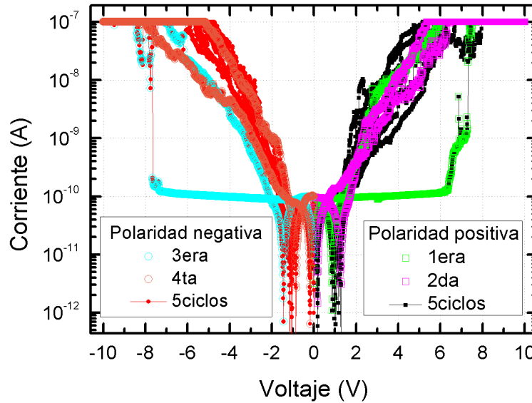
Figura 7.37: Módulo de la corriente en función del voltaje. Las excusiones sucesivas para cada polaridad demuestran la persistencia de los estados PLRS y NLRs .
