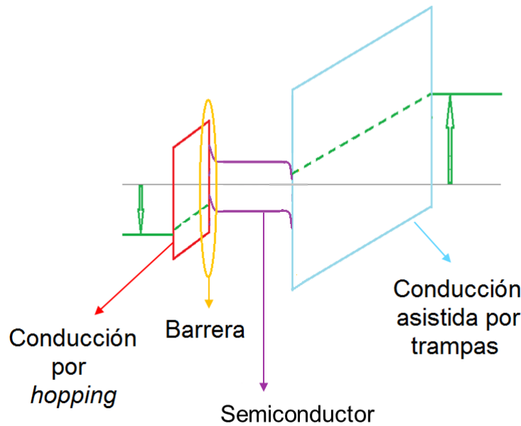
Figura 7.30: Diagrama de bandas atribuido al apilamiento bajo una condición de polarización negativa aplicada en el TE antes de producirse el evento de SET . Las líneas punteadas reflejarían el nivel habilitado, dentro de cada barrera representada por los óxidos SiO_{2-x} y HfO_{2-x} , por la presencia de impurezas en las respectivas capas.
