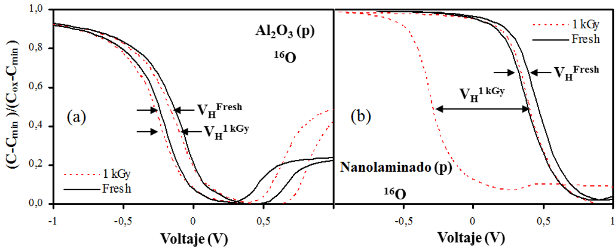
Figura 3.5: C - V normalizada de las estructuras irradiadas con iones de oxígeno. Los dieléctricos en cada caso son: (a) Al_2O_3 (b) NL , ambos sobre sustrato tipo p .
