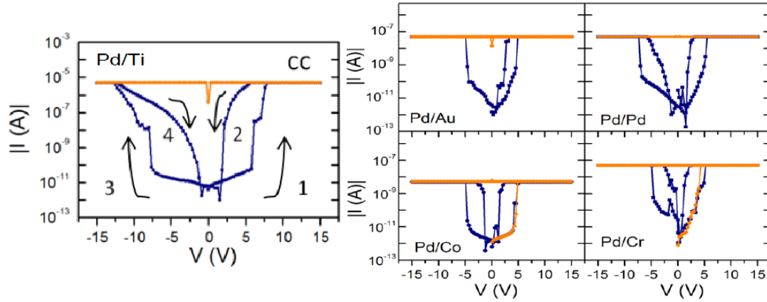
Figura 7.21: |I| – V de apilamientos con Pd como BE y los distintos metales depositados como TE : Cr , Au , Pd , Ti y Co , extraído de [53].
