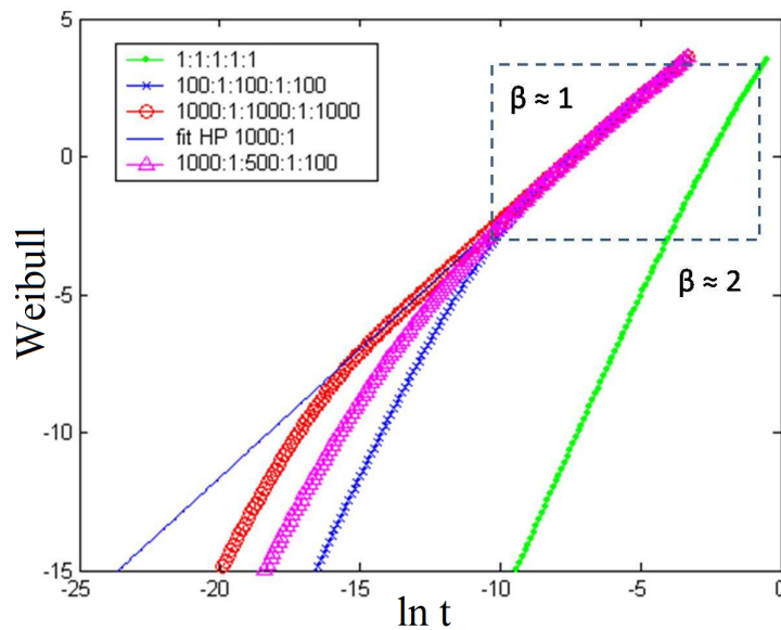
Figura 4.5: Modelo percolativo empleando 5 subcapas. Cada curva corresponde a distintas tasas de degradación ( A_1 : A_2 : A_3 : A_4 : A_5 ), véase el Apéndice C para una descripción de los parámetros. Todas ellas fueron generadas considerando \alpha = 0,38 [37].
