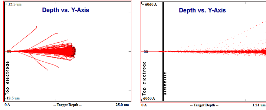
Figura 3.3: Simulación del recorrido de los iones de oxígeno O^{16} de 20 MeV al incidir en un apilamiento Al (200 nm) / Al_2O_3 (12 nm) / Si (500 \mu m ) efectuada con el código SRIM . Las líneas rojas identifican el paso de las partículas pesadas que, según puede verse, atraviesan las capas metálica ( Al ) y dieléctrica ( Al_2O_3 ) para implantarse en el semiconductor.
