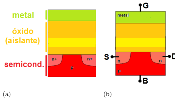
Figura 5.1: (a) Esquema de una memoria NROM en donde se destaca el apilamiento vertical MIS . (b) Representación de los electrodos accesibles externamente en la estructura.
