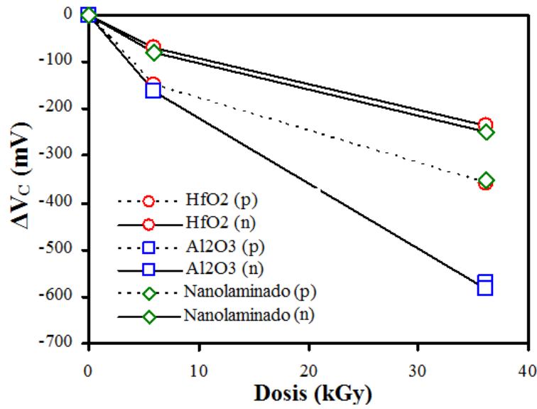
Figura 3.8: Evolución del voltaje para el que se alcanza la condición V_C en función de la dosis de radiación \gamma entregada.
