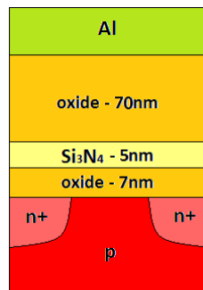
Figura 5.3: Detalle del apilamiento NROM empleado en este Capítulo. El laminado \text{SiO}_2/\text{Si}_3\text{N}_4/\text{SiO}_2 constituye el aislante de la estructura MIS . El nitruro es el material que actúa como pozo de potencial entre las barreras de \text{SiO}_2 , por la diferencia entre las bandas de conducción de la estructura.
