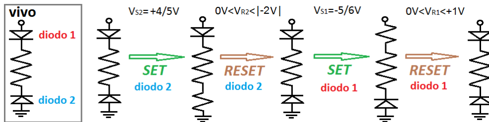
Figura 7.8: Modelo eléctrico propuesto para cada estado. Cada diodo es alternativamente reemplazado por una resistencia en lo que se denomina evento de SET . La operación de RESET , aunque inapreciable de la observación de la curva I - V , pudo ser comprobada en las mediciones de resistencia remanente presentadas en la Fig. 7.6.
