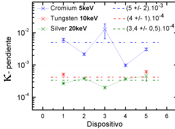
Figura 5.13: Tasa de degradación (definida como \kappa en la ec. 5.1) para 5 dispositivos de un mismo DIP , medidos en simultáneo con las mismas condiciones de polarización. Los valores \kappa fueron obtenidos individualmente empleando la rutina mencionada. Cada grupo de dispositivos sometidos a fotones de la misma energía se identifican con un mismo color.
