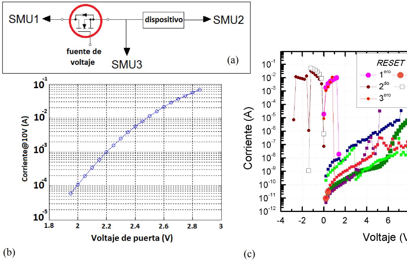
Figura 6.9: (a) Esquema de la conexión empleada en la configuración 1T 1R. (b) Curva de calibración del transistor empleado (2N 7000). La corriente máxima en el canal se controla mediante el voltaje aplicado en la puerta. (c) Módulo de la corriente en función del voltaje, I - V (aplicando V como estímulo), para las operaciones efectivas de SET y RESET de un dispositivo MgO-3 iii de la Tabla 6.1.
