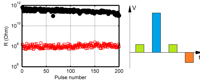
Figura 7.7: Resistencia remanente calculada para cada voltaje de lectura (esquemáticamente identificados en verde) aplicado entre las operaciones de escritura (en azul) y borrado (en naranja). En esta medición se emplean voltajes de lectura positivos con lo cual las resistencias corresponden a PHRS (en negro) y a PLRS (en rojo). De manera análoga para detectar NHRS y NLRS hubiese sido preciso emplear voltajes de lectura y SET negativos, mientras que el RESET hubiese requerido la aplicación de la polaridad contraria.
