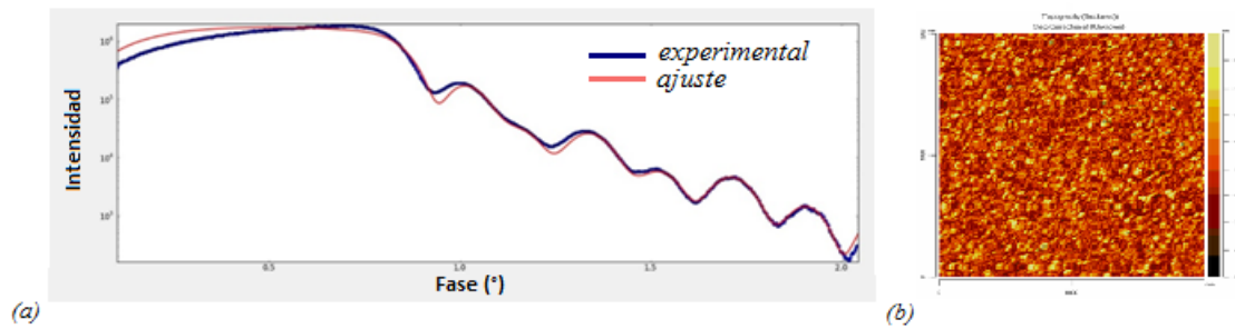
Figura 7.17: (a) Reflectividad de rayos X ( XRR ). La falta de periodicidad se debe a la multiplicidad de capas de materiales diferentes. (b) De la topografía efectuada con el microscopio de fuerza atómica se extrajo la medición de rugosidad necesaria para el ajuste de la señal en (a). Los parámetros empleados se presentan en la Tabla 7.1. La autora agradece a Alex Hardtdegen y Hehe Zhang del Forschungszentrum Jülich por las mediciones XRR y AFM , respectivamente.
