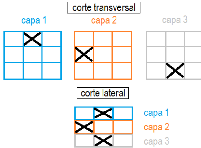
Figura C.1: La probabilidad de falla de un camino percolativo es menor que la de una columna de celdas apiladas, pues se considera que la conducción es posible aún cuando los elementos se contacten sólo por un extremo. Los recuadros con cruces ejemplifican las celdas defectuosas que constituyen el camino percolativo.
