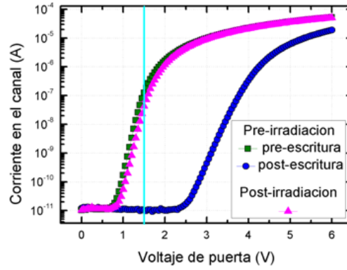
Figura 5.10: Corriente en el canal ( I_{DS} ) en función del voltaje de puerta ( V_G ) para los casos programado (pre irradiación) y post irradiación. Dado que la interpretación de lo que sucede en el nitruro se efectúa de manera indirecta, a través de la lectura en el canal, no es posible discernir entre la pérdida de los electrones almacenados y el atrapamiento de carga positiva (que compense el efecto de los electrones).
