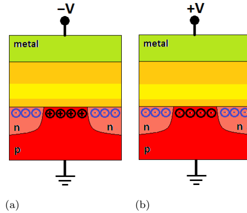
Figura 5.2: (a) Estructura NROM en la condición en que el semiconductor se halla en acumulación. (b) Estructura NROM en la condición en que el semiconductor se halla en inversión.
