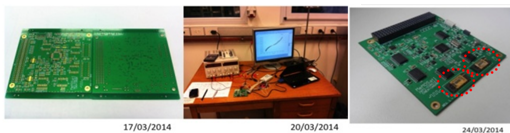
Figura D.1: Fotografías de la plaqueta en su fase de diseño, del set up empleado para la caracterización de las memorias una vez montadas en la misma y de la plaqueta terminada (en donde se destacan las ubicaciones de las estructuras ReRAM ). Los distintos pasos fueron llevados a cabo en su totalidad por los integrantes del Proyecto MeMOSat (fotografías gentileza de Fernando Gómez Marlasca).
