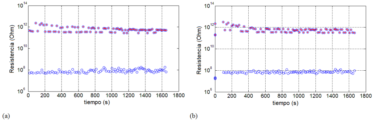
Figura 7.16: Lecturas sucesivas de la resistencia en cada estado ( PHRS y PLRS ) antes (a) y después (b) de la irradiación.
