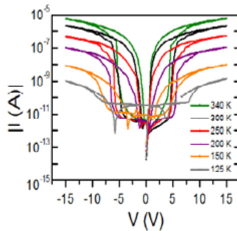
Figura 7.26: Módulo de la corriente en función del voltaje para distintas temperaturas de medición, extraído de [53].
