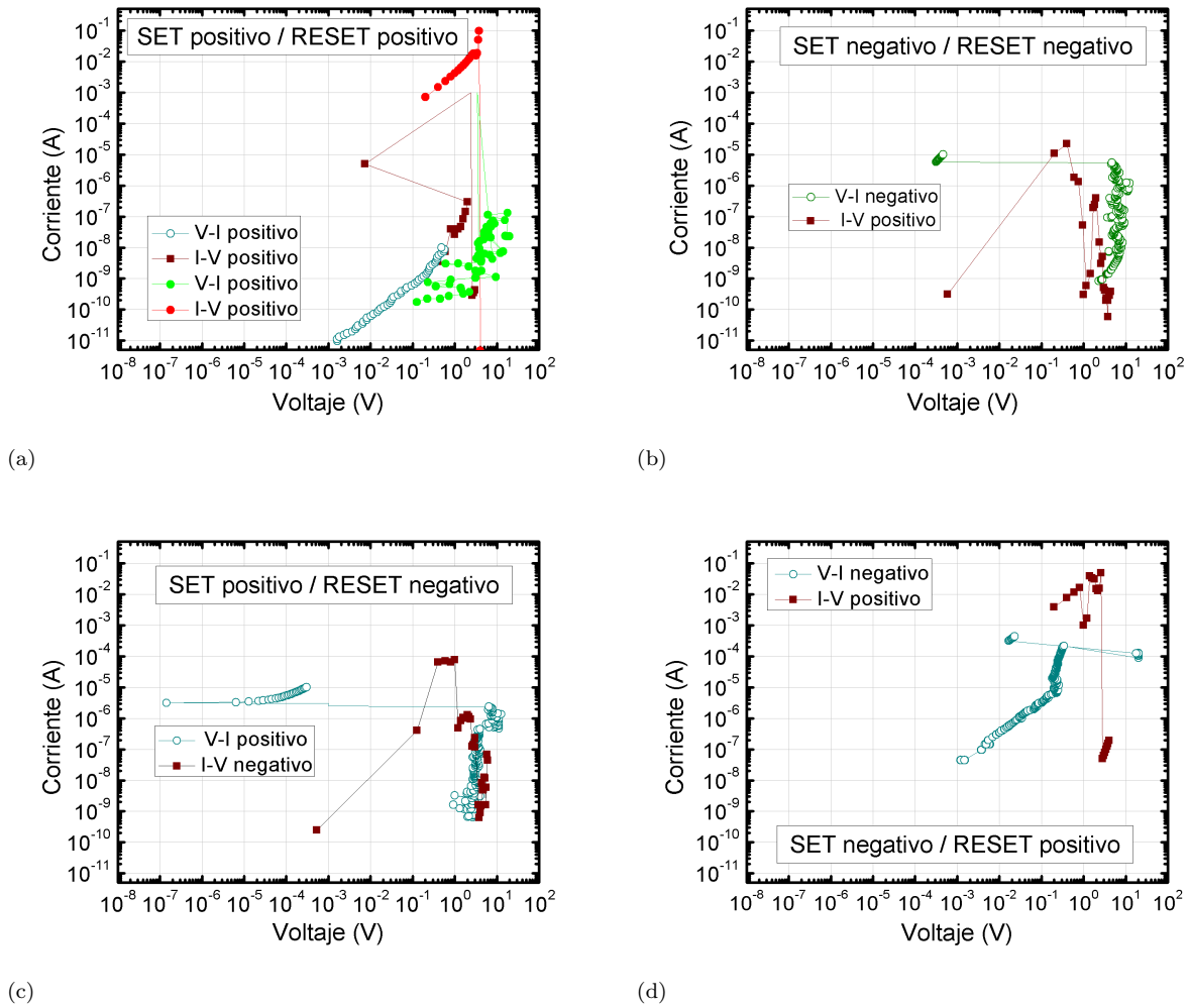
Figura 6.8: Operaciones de escritura y borrado con las distintas combinaciones de polaridad posible: (a) SET positivo - RESET positivo, (b) SET negativo - RESET negativo, (c) SET positivo - RESET negativo y (d) SET negativo - RESET positivo. Esto ilustra el carácter apolar de la conmutación analizada. Los ejes de corriente y voltaje están expresados en módulo.
