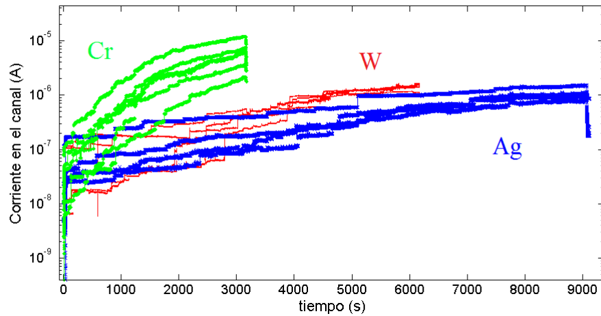
Figura 5.14: Corriente en el canal en función del tiempo de exposición a la radiación (dispositivos prístinos). Los trazos de color verde corresponden a la irradiación con Cr , los azules a Ag y los rojos al W .
