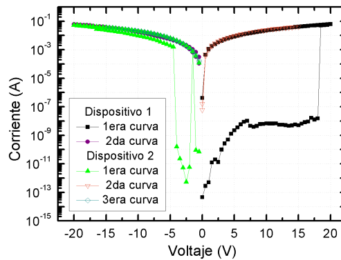
Figura 7.23: Módulo de la corriente en función del voltaje para dos dispositivos con estructura Pd/Co/HfO_2/Si . Las excursiones sucesivas demuestran ausencia de la propiedad denominada autolimitación de corriente.
