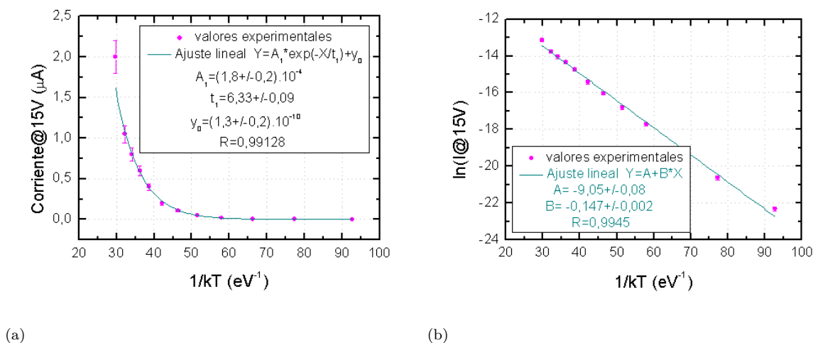
Figura 7.28: (a) Corriente en función de la inversa de la temperatura. El ajuste exponencial demuestra un buen acuerdo con los datos experimentales. (b) Logaritmo de la corriente en función de la inversa de la temperatura (a la manera de un gráfico de Arrhenius). El ajuste lineal, equivalente al ajuste exponencial en (a), demuestra la correlación entre el parámetro I@ + 15 V con respecto a T .
