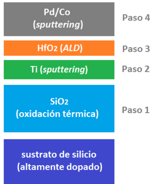
Figura 7.1: Esquema de la sucesión de pasos seguidos para la obtención del apilamiento final.
