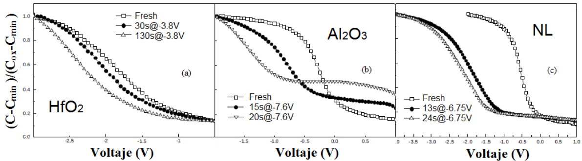
Figura 3.11: C - V antes, durante y después de mediciones de estrés eléctrico. La comparación entre ellas demuestra que las mediciones en sí mismas producen cambios en la composición del aislante.
