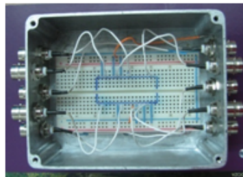
Figura 5.9: Fotografía del adaptador empleado para extraer conectores coaxiales a partir de los pines del DIP .
