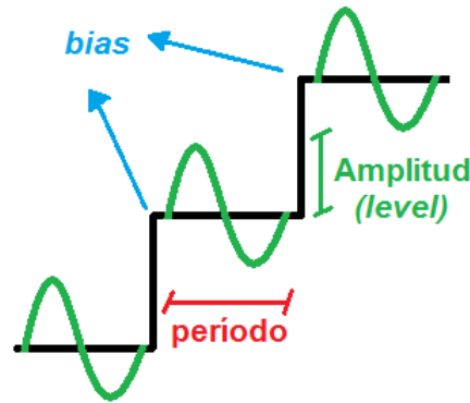
Figura 2.2: Esquema del estímulo que se aplica al medirse capacidad. Quedan de manifiesto los parámetros fundamentales a considerar al efectuar dicha medición.
