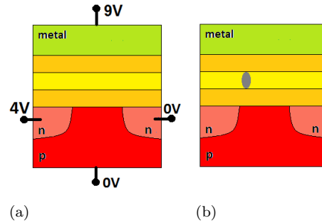
Figura 5.5: (a) Voltajes estipulados para la operación de escritura de un dato. (b) Esquema representando la carga acumulada en el nitruro.
