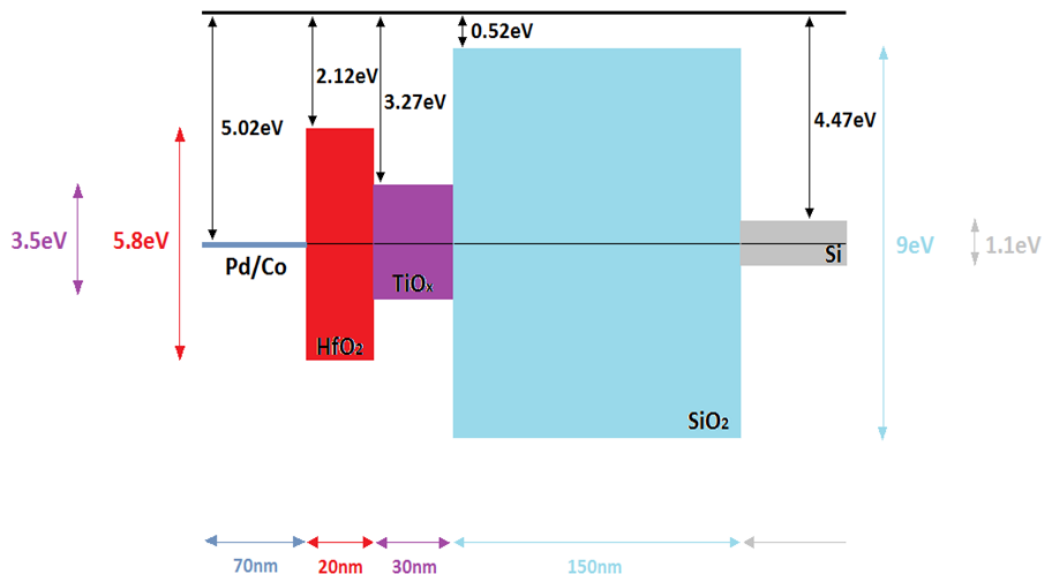
Figura 7.29: Diagrama de bandas para el dieléctrico laminado con que se cuenta (véase la Fig. 7.19). Las energías de ionización y de banda prohibida corresponden a los materiales estequiométricos, se usan aquí como valores de referencia.
