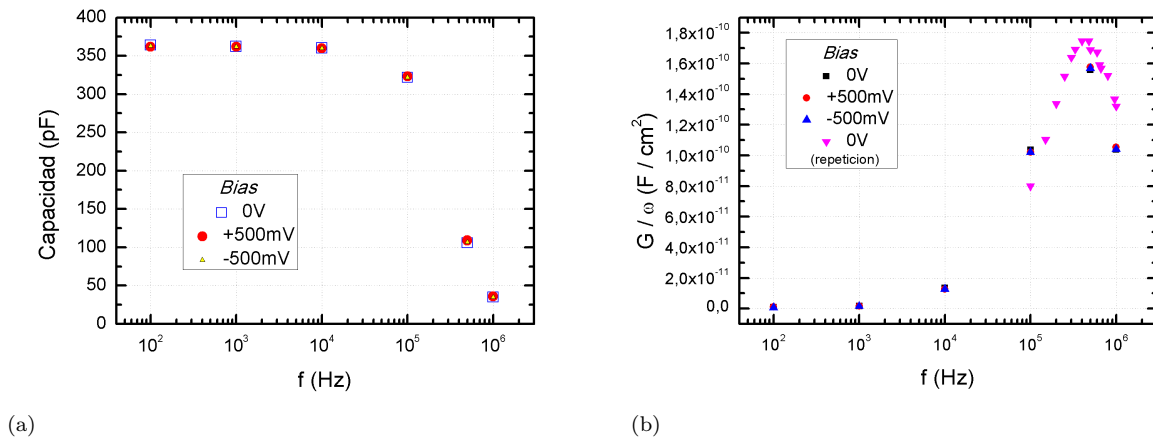
Figura 7.24: (a) Capacidad en función de la frecuencia medido en la estructura Pd/Co/HfO_2/Si . (b) \frac{G}{\omega} en función del logaritmo de la frecuencia.
