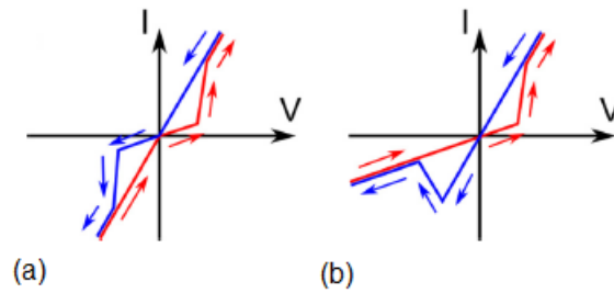
Figura 7.3: Esquema de curvas I - V (a) non crossing y (b) crossing . Esta clasificación corresponde a la observación de la curva I - V con los signos correspondientes a cada polaridad (compárese con la Fig. 7.2 (b)).
