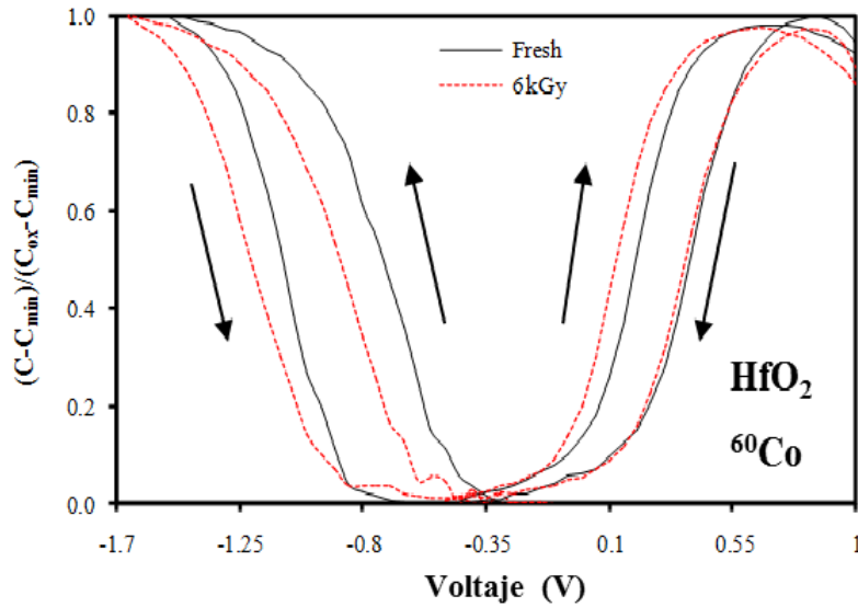
Figura 3.7: C - V de una estructura basada en HfO_2 irradiada con fotones \gamma ( Co^{60} ).
