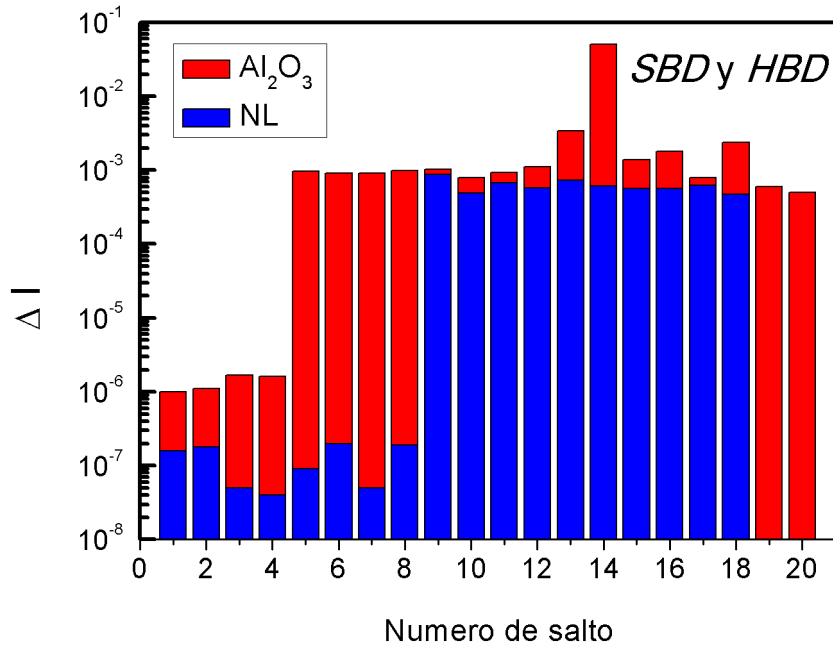
Figura 4.7: Gráfico de barras para los sucesivos incrementos de corriente registrados a un V fijo de la lectura I - V . Puede verse que durante el régimen SBD , los saltos atribuidos a la alúmina y al NL se distinguen mas no en el régimen HBD .
