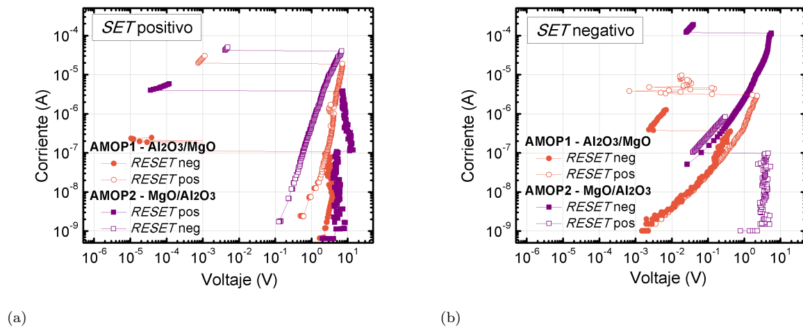
Figura 6.11: Curvas de corriente en función del voltaje. Se presentan operaciones de SET efectuadas con polaridades positiva (a) y negativa (b). La comparación radica en la polaridad empleada para la operación de RESET inmediata anterior. El estímulo empleado, en todos los casos, fue de corriente. El tipo de representación se mantuvo para facilitar la lectura y comparación de los gráficos.
