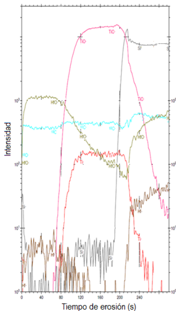
Figura 7.18: Materiales desprendidos de la muestra en función del tiempo de erosión (perfil SIMS ). La comparación entre las señales refleja la cantidad relativa de elementos en las sucesivas capas pero no permite extraer la estequiometría, a menos que se cuente con una muestra patrón. La autora agradece a Aleksei Savenko del Forschungszentrum Jülich por la medición SIMS .
