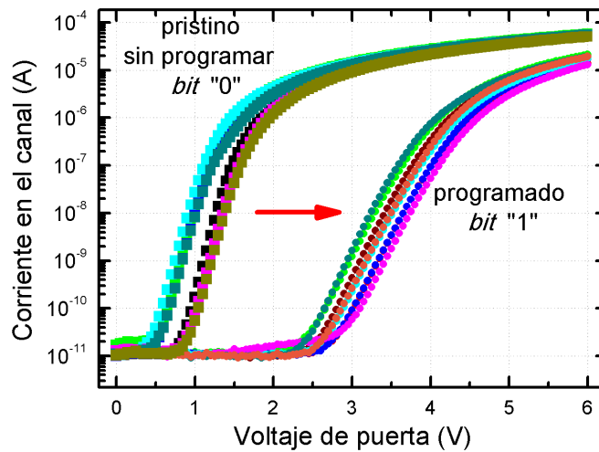
Figura 5.7: Corriente en el canal ( I_{SD} ) medida en función del voltaje de puerta ( V_G ) para distintos dispositivos de un mismo DIP en estado programado. Si se compara con la Fig. 5.6 (b) puede verse que, a medida que se produce la pérdida de la carga, la corriente medida bajo una misma tensión deberá ir en aumento. Las curvas ejemplifican la dispersión posible. El voltaje destacado corresponde al punto de trabajo que se tomará como referencia para observar la evolución de la carga atrapada.
