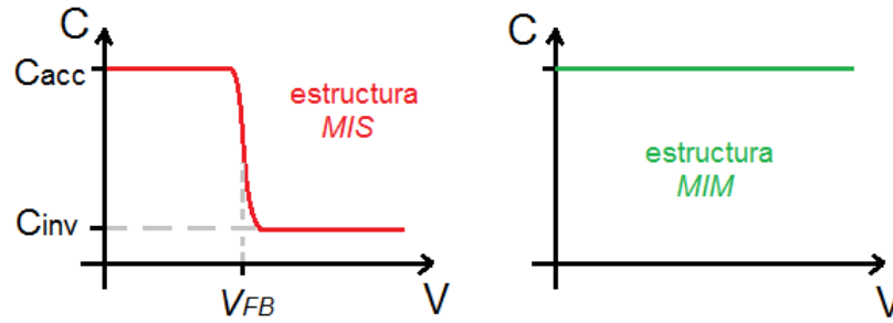
Figura 1.1: Dependencia típica de capacidad en función del voltaje para los dos tipos de estructura tratados en la Tesis, MIS y MIM .
