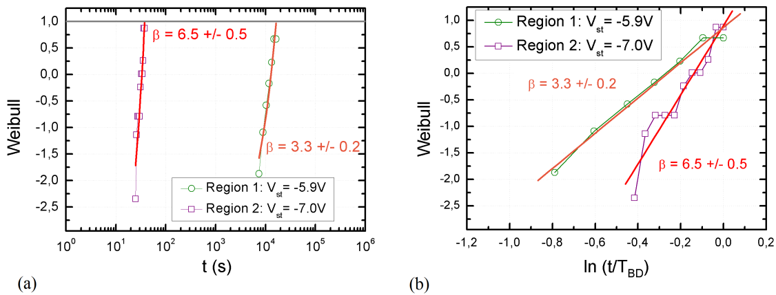
Figura 4.4: (a) W vs. \log_{10}t (b) W vs. \ln(\frac{t}{T_{BD}}) para estructuras basadas en el dieléctrico NL . W se define en función de los datos experimentales en la ec. 4.7 (correspondientes a unos 50 dispositivos). La expresión W empleada para los ajustes considera la simplificación expuesta en la Fig. 4.3.
