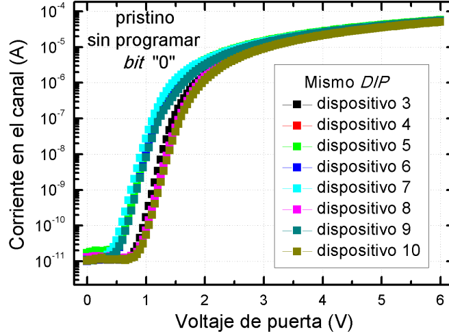
Figura 5.4: Corriente que circula en el canal ( I_{SD} ) en función del voltaje aplicado en la puerta ( V_G ) para distintos dispositivos. La superposición de curvas refleja la dispersión entre dispositivos.
