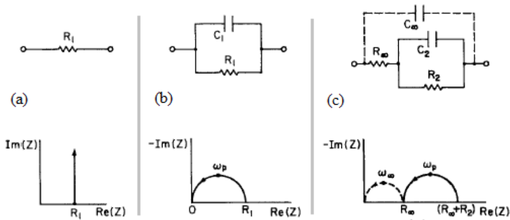
Figura 2.5: Diagramas Cole-Cole para los arreglos detallados en cada caso (extraído de [4]).
