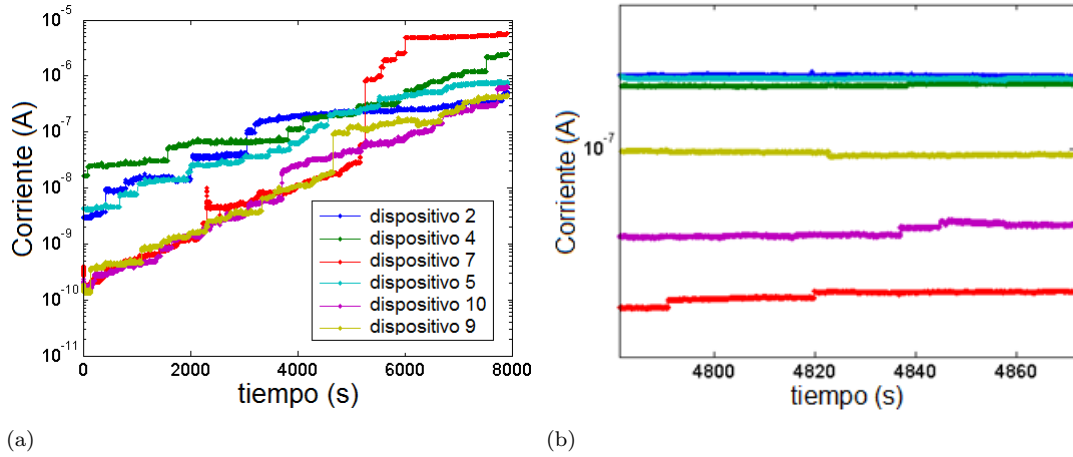
Figura 5.15: (a) Corriente en función del tiempo medida para múltiples dispositivos en simultáneo. (b) Detalle de la medición mostrada en (a).
