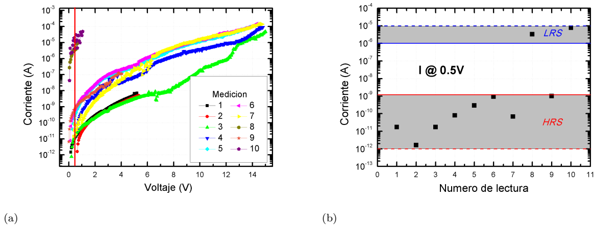
Figura 6.6: (a) Curvas I - V sucesivas medidas en un mismo dispositivo. (b) Lecturas a 500mV del estado remanente luego de cada I - V mostrada en (a). La dispersión en los niveles de corriente manifiesta la presencia de estados intermedios entre los que se mostraban en la Fig. 6.4.
