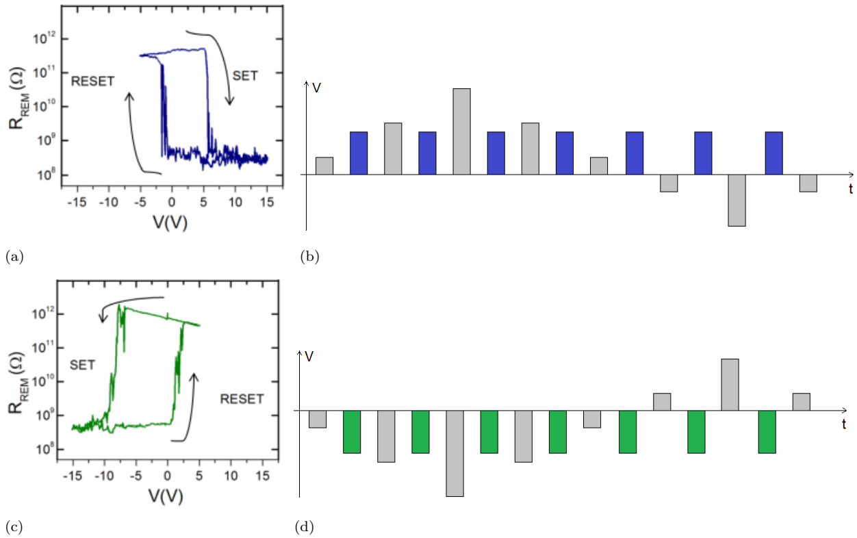
Figura 7.6: Resistencia remanente en función del estímulo inmediato anterior [53]. La resistencia remanente se calcula a partir de la medición de lectura (en azul en (b) y en verde en (d)) pero se grafica en función del estímulo inmediato anterior de la rampa dinámica (representados en gris). La polaridad del voltaje de lectura (positivo en (a) y negativo en (c)) permite identificar alternativamente cada una de las dos junturas.
