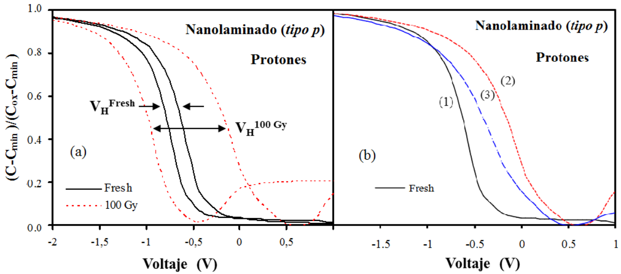
Figura 3.6: C - V de las estructuras NL irradiadas con protones. (a) Curvas de IDA y VUELTA para apreciar la variación en la histéresis. (b) Curvas de IDA para los casos: prístino (1) e irradiado (2) y (3). Luego de la segunda irradiación, curva etiquetada como (3), el sistema parece restituirse parcialmente.
