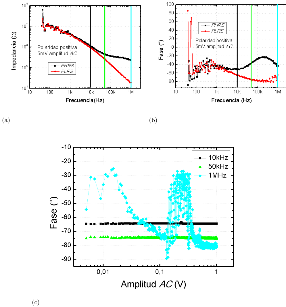
Figura 7.13: (a) |Z| y (b) \psi en función de la frecuencia, aplicando +4V de bias con 5mV de amplitud AC) (c) Cambio de HRS a LRS con el aumento de la amplitud de AC.
