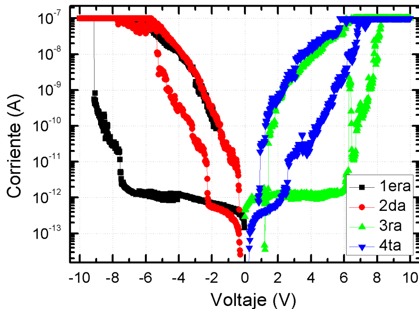
Figura 7.36: Módulo de la corriente en función del voltaje medido en un dispositivo de la muestra FZJ 10A .
