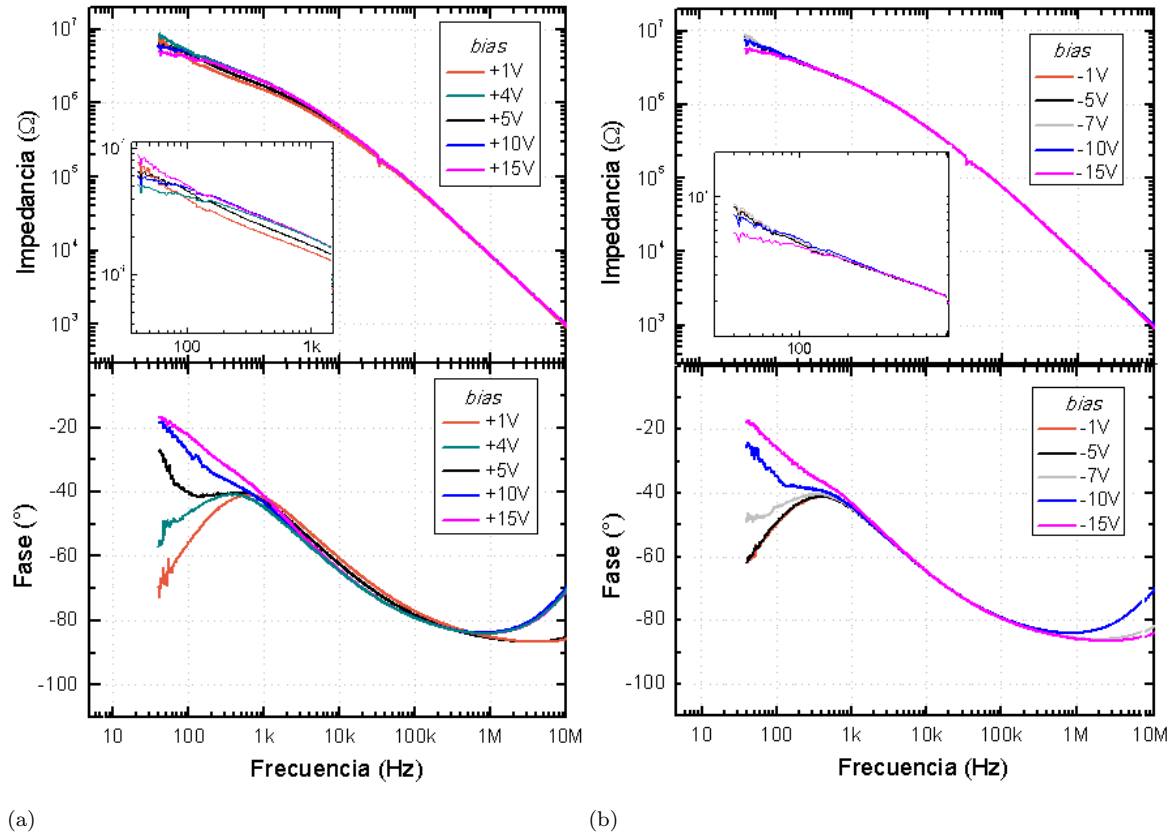
Figura 7.12: Módulo ( |Z| ) y fase ( \psi ) de la impedancia en función de la frecuencia para distintos bias de polaridades (a) positivas y (b) negativas. Todas las mediciones fueron efectuadas con una amplitud de 500 mV.
