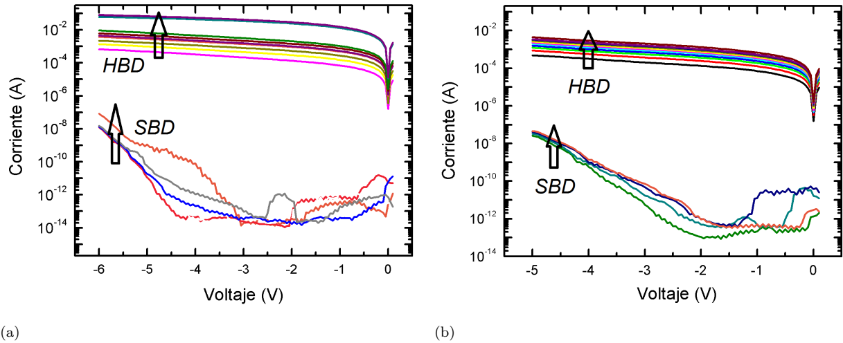
Figura 4.6: Sucesión de curvas |I| - V registradas después de cada evento identificado en la medición CVS asociada para una estructura basada en (a) Al_2O_3 y (b) NL .
