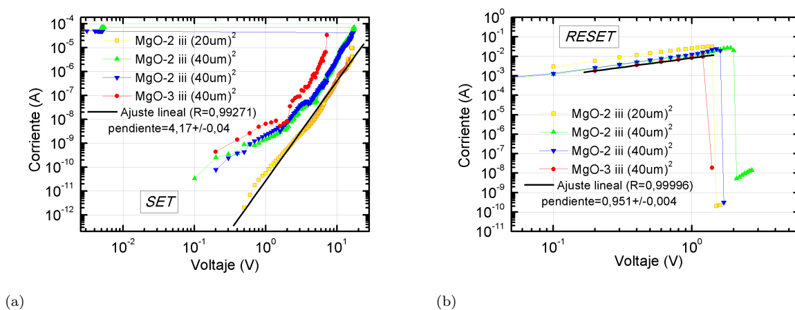
Figura 6.7: Operaciones de (a) SET ( HRS \rightarrow LRS ) y (b) RESET ( LRS \rightarrow HRS ) para dispositivos de diferentes muestras. Las designaciones corresponden a la Tabla 6.1. La representación doble logarítmica permite identificar mecanismos de conducción posibles.
