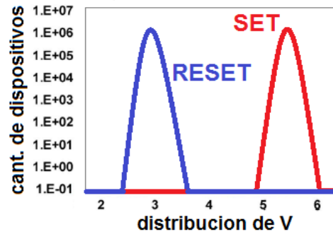
Figura 6.5: Esquema de la dispersión esperada para los voltajes de SET (escritura) y RESET (borrado). La diferencia entre el mínimo valor de SET y el máximo de RESET es lo que se denomina ventana y permite distinguir los estímulos necesarios para observar cada una de las operaciones.
