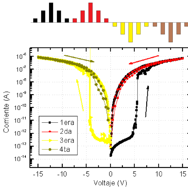
Figura 7.5: Excursiones sucesivas para una misma polaridad (protocolo de rampa pulsada). Se aprecia que el hecho de alcanzar los 0\text{ V} no supone la pérdida del estado alcanzado. Los colores empleados en la representación de las curvas se condicen con el protocolo indicado con el mismo color en el detalle superior.
