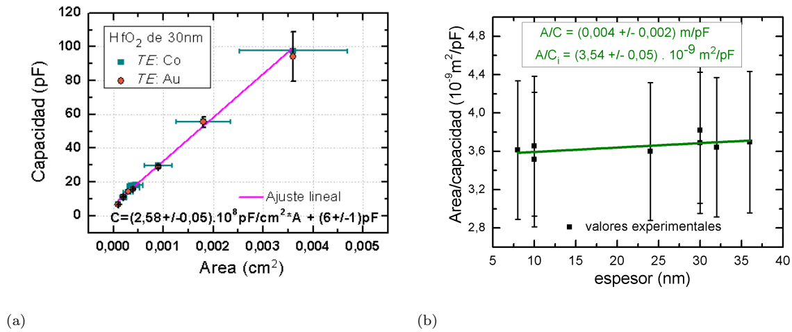
Figura 7.20: (a) Capacidad en función del área del dispositivo. Las barras de error horizontales provienen de la comparación del área nominal con el área efectiva de los electrodos (análisis efectuado en base a fotografías tomadas con un microscopio óptico). (b) Capacidad en función del espesor del dispositivo. Las mediciones se efectuaron a 500 kHz, con una amplitud AC de 50 mV y un bias de 0 V. Las barras de error en la medición de capacidad provienen de las fluctuaciones identificadas en la lectura a lo largo del tiempo. Los parámetros \frac{A}{C} y \frac{A}{C_i} corresponden a la pendiente y ordenada, respectivamente, del ajuste lineal.
