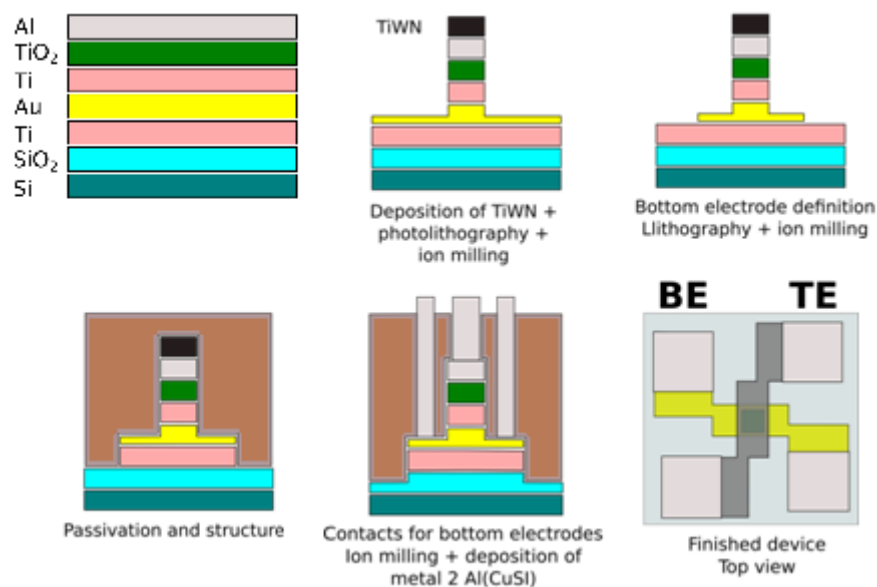
Figura A.4: Pasos sucesivos para la determinación de electrodos post-deposición de las capas de los distintos materiales (gentileza de Mariano Barella).
