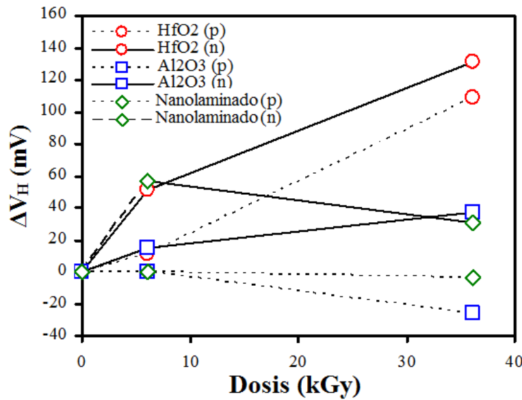
Figura 3.9: Evolución de la histéresis entre las curvas de IDA y VUELTA ( \Delta V_H ) en función de la dosis de radiación \gamma entregada.
