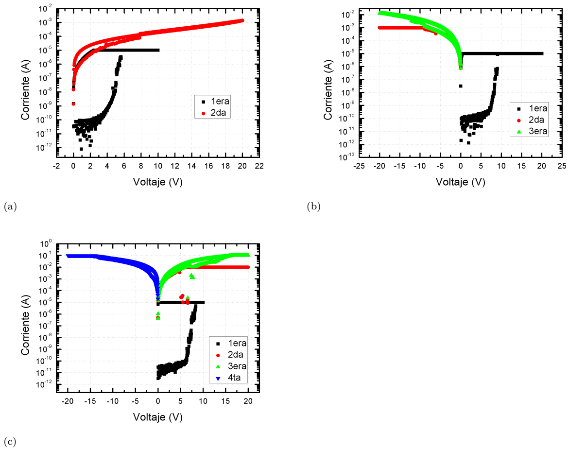
Figura 7.33: |I| - V de las muestras (a) FZJ 7A , (b) FZJ 9A y (c) FZJ 10A , todas ellas contactando el BE mediante un scratch .
