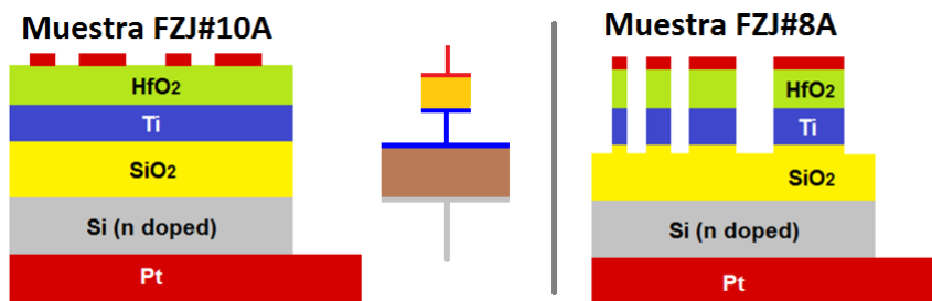
Figura 7.38: La comparación entre los capacitores determinados por el proceso de fabricación de la estructura manifiesta la necesidad de efectuar el patterning hasta aislar los dispositivos mutuamente. De otro modo, la persistencia de la capa de \text{Ti} metálica hubiera impedido el estudio de los cambios en la capa de \text{HfO}_2 .
