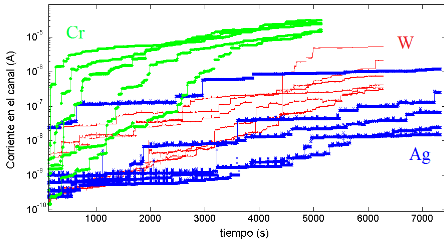
Figura 5.12: Corriente en el canal ( I_{SD} ) en función del tiempo de exposición a la radiación (dispositivos programados). Los trazos de color verde corresponden a la irradiación con Cr , los azules a Ag y los rojos al W .
