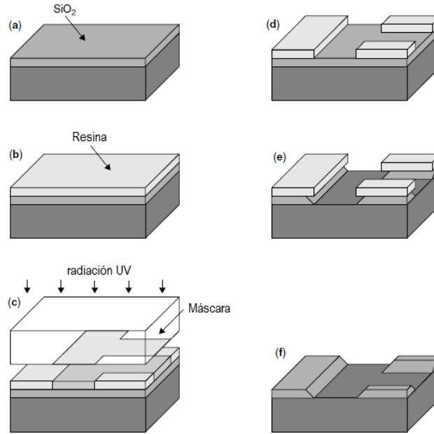
Figura A.1: Esquema de la exposición de una superficie a una fuente de luz mediante el empleo de una máscara (extraído de [5]).
