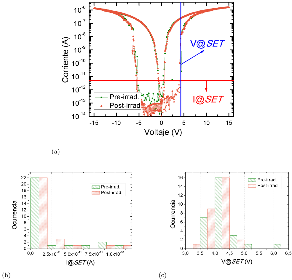
Figura 7.15: (a) Corriente en función del voltaje pre y post irradiación O^{16} de 20 MeV, dosis de 3 \cdot 10^{12} \frac{\text{iones}}{\text{cm}^2} . Los parámetros: corriente a la que se desencadena el SET ( I@SET ) y voltaje al que se aprecia la conmutación ( V@SET ) fueron analizados estadísticamente para todos los dispositivos irradiados (histogramas (b) y (c), respectivamente). Los bines de cada distribución fueron desfasados la mitad del ancho de cada uno para poder visualizar la ocurrencia de cada valor.
