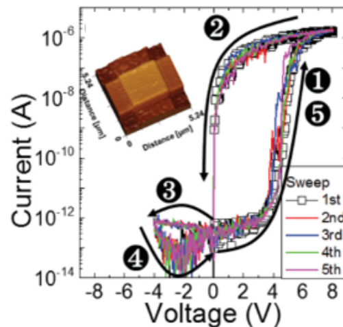
Figura 7.31: Antecedente de conmutación bipolar con características eléctricas similares a las de la Fig. 7.2 extraído de [68]. La coincidencia con la estructura del trabajo referido radicaría en la presencia de una interfaz entre HfO_{2-x} y Ti presumiblemente oxidado a causa del proceso ALD posterior.
