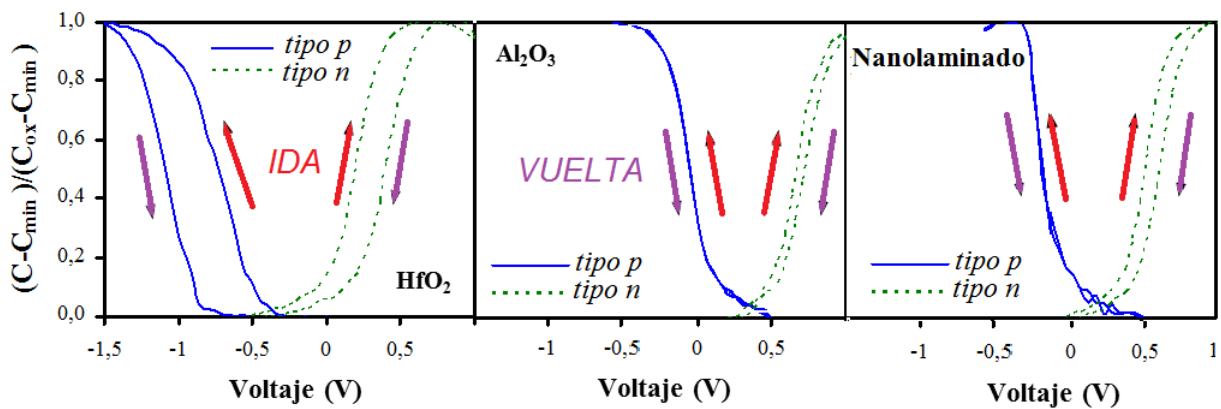
Figura 3.2: Capacidad en función del voltaje ( C - V ) medida en estructuras con los tres tipos de dieléctrico ( HfO_2 , Al_2O_3 y NL ) para los dos tipos de sustrato.
