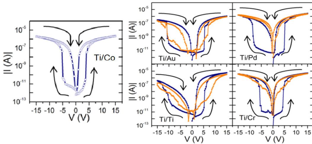
Figura 7.22: |I| – V de apilamientos con Ti como BE y los distintos metales depositados como TE : Cr , Au , Pd , Ti y Co , extraído de [53].
