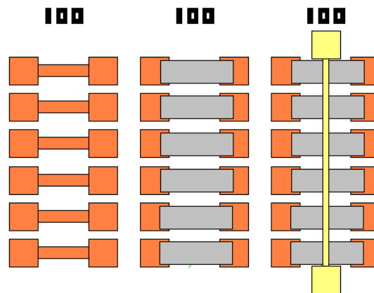
Figura A.3: Esquema de la superficies luego de las sucesivas fotolitografías. En el primer paso se determinan los electrodos inferiores. A continuación se delimita el área en que se deposita el dieléctrico y finalmente se definen los electrodos superiores.
