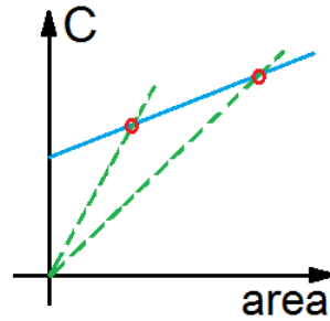
Figura 2.4: Capacidad en función del espesor de un dieléctrico que no es el único material presente en la estructura capacitiva.
