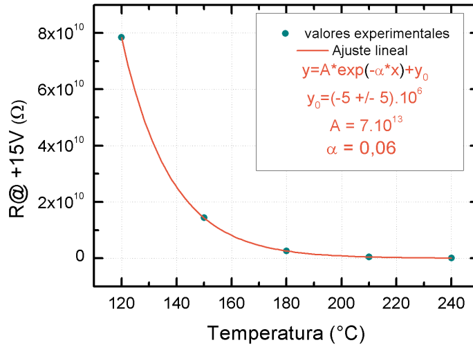
Figura 7.27: Resistencia medida a +15V en función de la temperatura de medición (extraído de [53]). El ajuste satisfactorio logrado con una función exponencial sugiere un comportamiento semiconductor.
