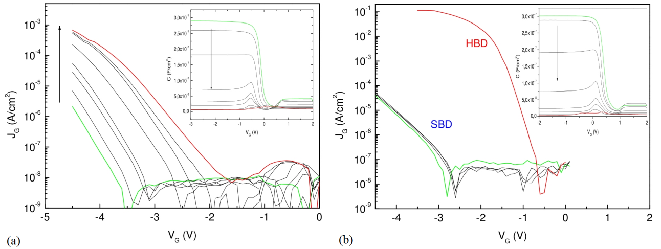
Figura 3.4: Densidad de corriente en función del voltaje. Mediciones efectuadas a intervalos regulares de dosis entregada en estructuras con Al_2O_3 (a) y NL (b) como dieléctricos (ambos sobre sustrato tipo p ) irradiadas con iones de oxígeno.
