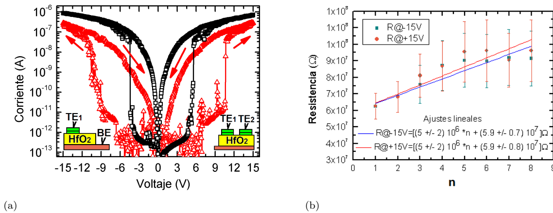
Figura 7.10: (a) Comparación de las curvas I - V medidas en un único dispositivo (conexión transversal) y entre electrodos superiores (conexión serie). (b) R@ + 15 V y R@ - 15 V en función del número de electrodo vecino ( n = 1 significa que la señal se aplica entre un electrodo y el primer vecino: d = 200 \mu m ).
