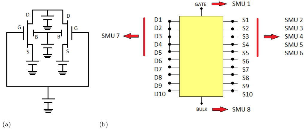
Figura 5.8: (a) Esquema de la conexión empleada para el registro de la señal en varios dispositivos durante el mismo tiro de radiación. Nótese que los D_i están cortocircuitados entre sí y que los contactos G y B son únicos para todos los canales. (b) Esquema de la visualización del DIP con sus distintos contactos disponibles.
