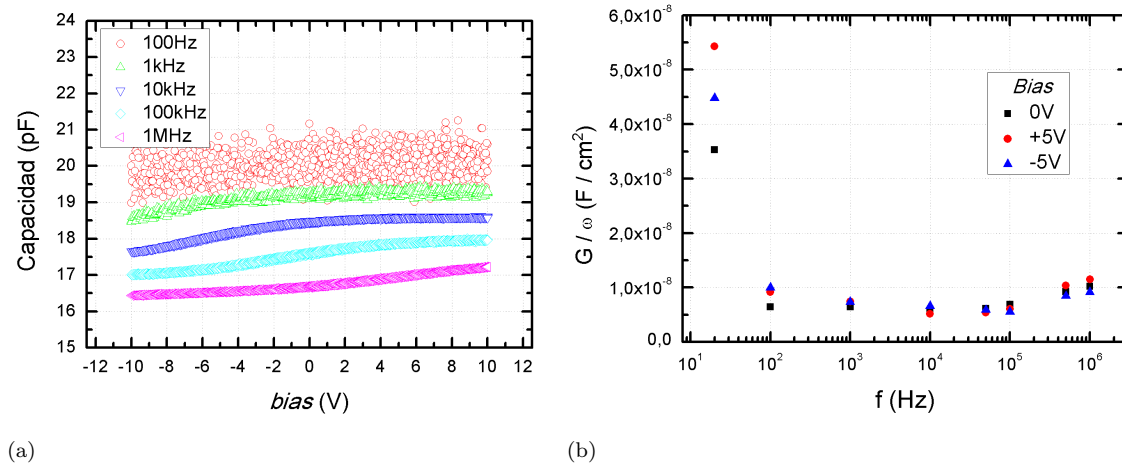
Figura 7.34: (a) Capacidad en función del voltaje de polarización ( bias ) medida a distintas frecuencias en la muestra FZJ 13A en un dispositivo de 5 \cdot 10^{-8}m^2 de área. (b) \frac{G}{\omega} en función del logaritmo de la frecuencia. La ausencia de un pico en dicha representación descarta la predominancia de un tiempo característico de atrapamiento de carga.
