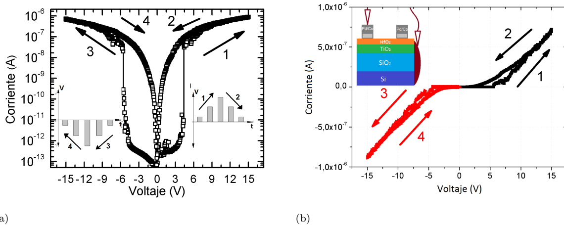
Figura 7.2: (a) Módulo de la corriente (logarítmica) en función del voltaje, medida con protocolo de rampa de pulsos. (b) Corriente en función del voltaje (escala lineal). Puede apreciarse el comportamiento designado como non crossing .
