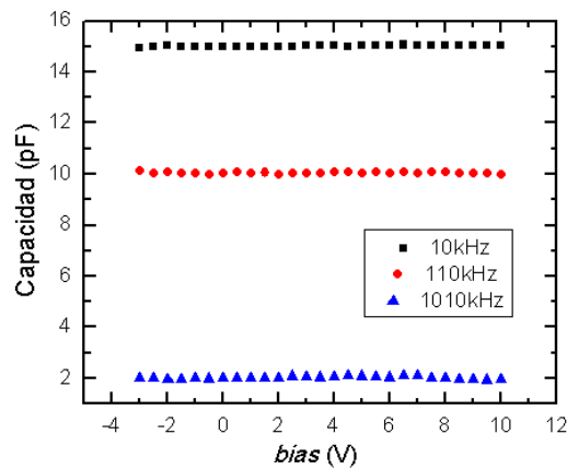
Figura 7.11: Capacidad en función del voltaje de polarización ( bias ) adquiridas con una señal AC de las frecuencias especificadas y una amplitud AC de 100 mV .
