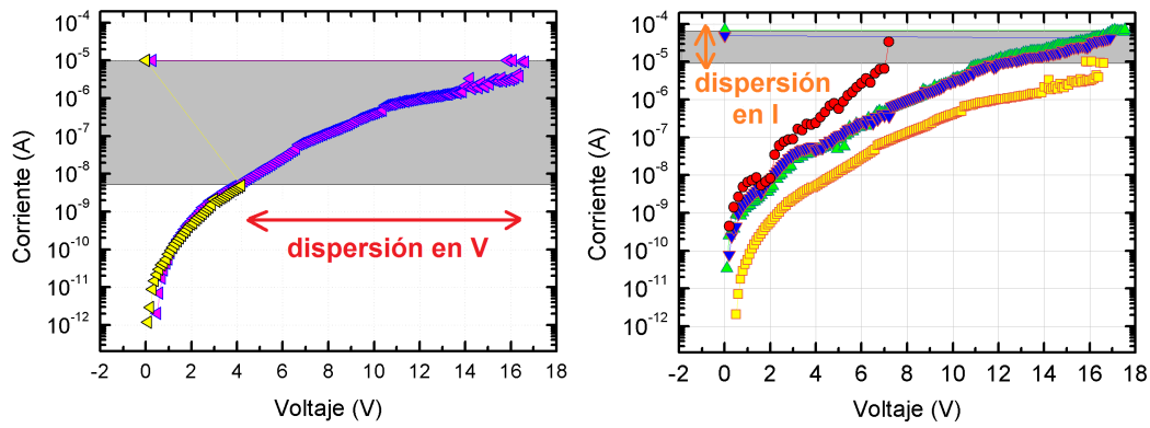
Figura 6.10: Curvas de SET efectuadas empleando (a) voltaje y (b) corriente como estímulo, respectivamente, aunque ambas se grafican como I-V con fines comparativos. El reemplazo del estímulo V por el de I para la operación de SET refleja el impacto que la alternancia de protocolos produce en la repetibilidad de las condiciones.
