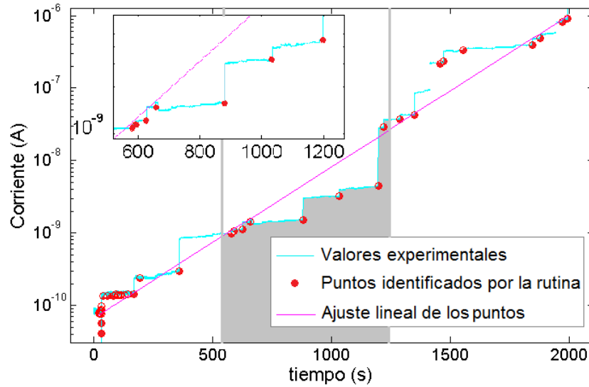
Figura 5.11: Corriente en el canal ( I_{SD} ) en función del tiempo de exposición a la radiación para la condición V_G = 1,5V con V_B = V_D = 0V . El inset corresponde a la región resaltada en gris.
