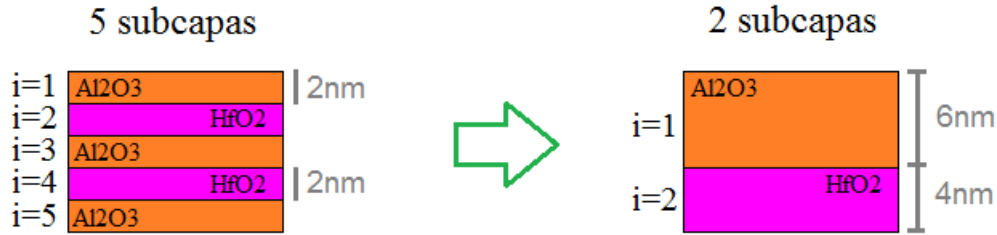
Figura 4.3: Simplificación del NL fabricado (5 subcapas: 3 de Al_2O_3 de 2 nm cada una y 2 de HfO_2 de 2 nm cada una) mediante un apilamiento compuesto por sólo dos subcapas: 6 nm de Al_2O_3 y 4 nm de HfO_2 .
