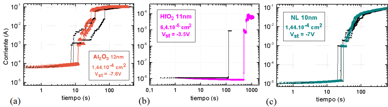
Figura 4.1: Corriente en función del tiempo (mediciones de estrés eléctrico) para los aislantes (a) Al_2O_3 ( CVS@-7,5V ) (b) HfO_2 ( CVS@-3,5V ) (c) NL ( CVS@-7V ). En cada caso se especifica la condición de polarización empleada, el espesor del dieléctrico y el área de los dispositivos estresados.
