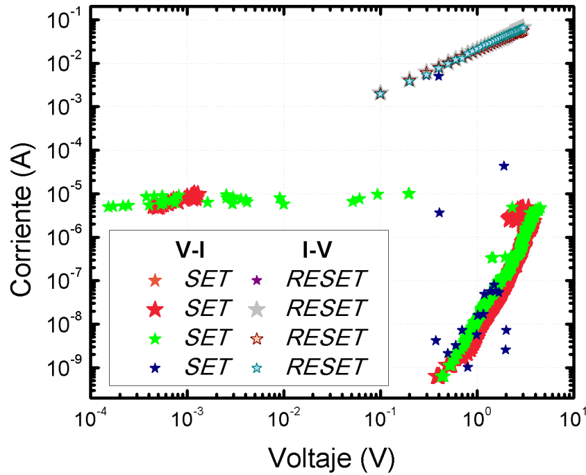
Figura 6.12: |I| - V para un dispositivo de la muestra AMOP1 . Las operaciones de SET se efectuaron estimulando en corriente, mientras que en las de RESET se estimuló en voltaje.
