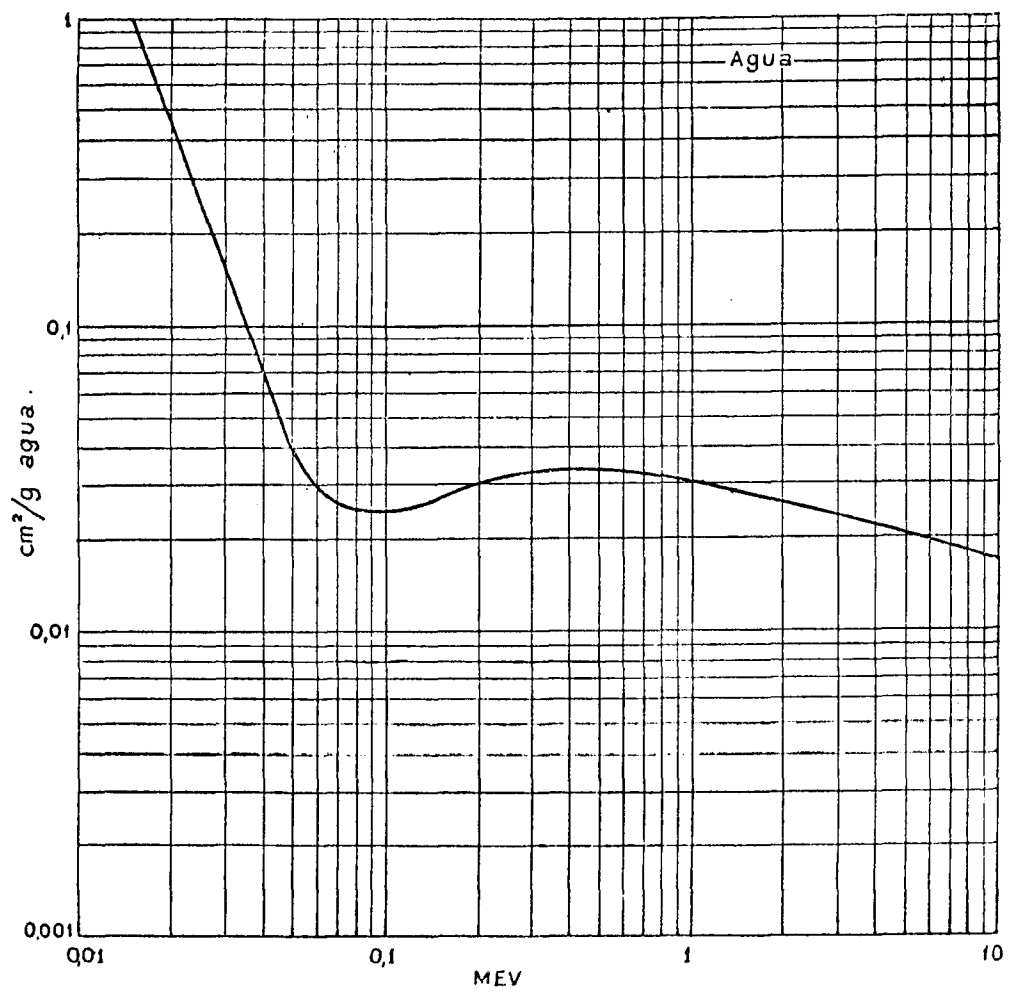
Fig. 22' Coeficiente de absorción másico para agua
