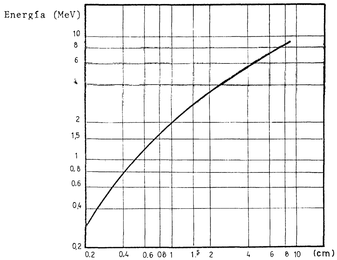
FIG. 6 - Alcance Medio Para Partículas \alpha En Aire
