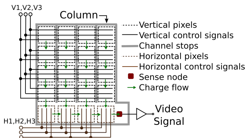
Figura 1.2: Estructura de un CCD bidimensional de 4x4 píxeles
