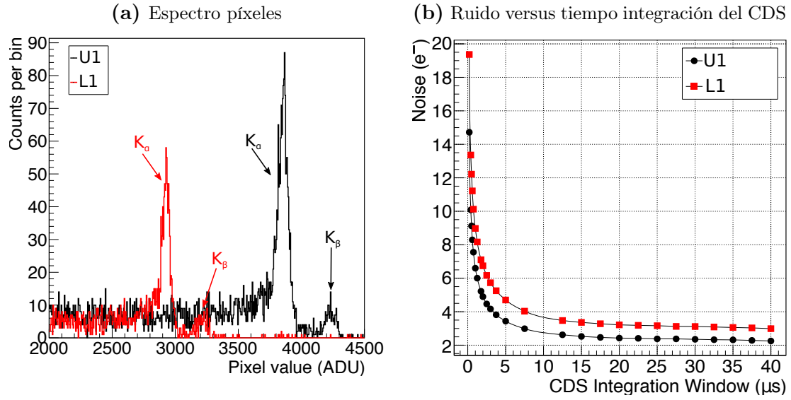
Figura 5.10: Figura (a): espectro en el rango del rayo X K_\alpha (5.9 keV) de la fuente ^{55}\text{Fe} . Figura (b): ruido a diferentes tiempos de integración. El cuadrante U1 tiene mayor ganancia y menor ruido debido a que el área del SN es menor. para un tiempo de integración de 2.5 \mu s la ganancia obtenida con U1 es de 2.46 \text{ ADU}/e^- y el ruido es de 4.47 e^- .
