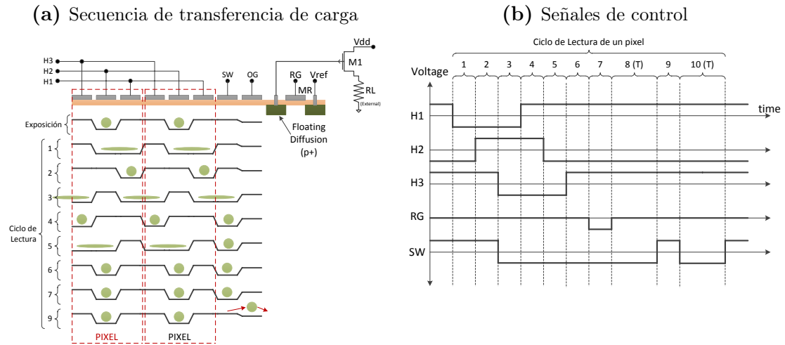
Figura 2.8: Secuencia de transferencia de carga de los píxeles verticales a horizontal, la burbuja verde representa el paquete de carga del pixel.
