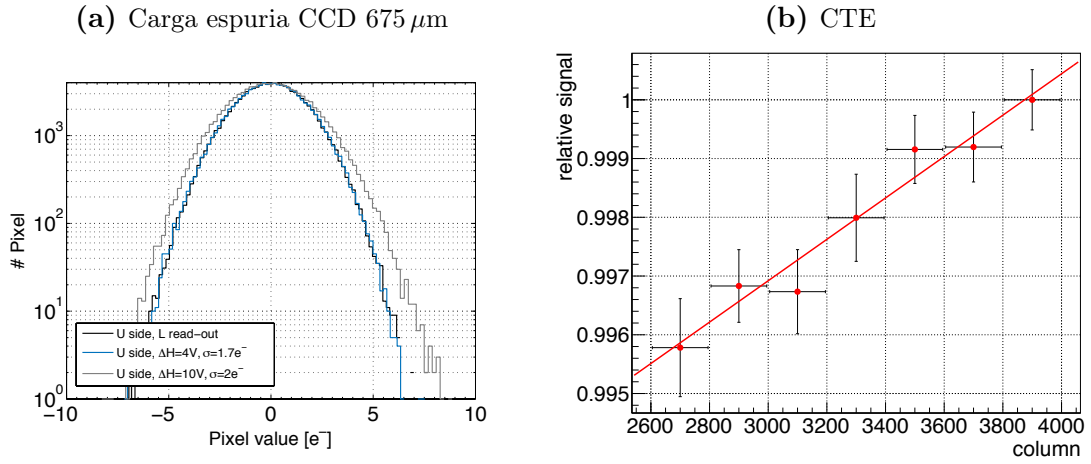
Figura 4.3: Ruido electrónico (histograma en negro) y ruido total para dos conjuntos de voltajes de las señales de control de un CCD fully-depleted de 675\mu m . Para el conjunto de voltajes optimizados de la tabla 4.1 el ruido total medido es igual que el ruido electrónico del canal. En (b) se muestra la medición de CTE: 98.63 %, se observa la pérdida de señal entre la primer y última columna leída. Solamente se expuso una fracción de columnas, porque en el arreglo experimental las restantes estaban cubiertas por el cable flexible del CCD.
