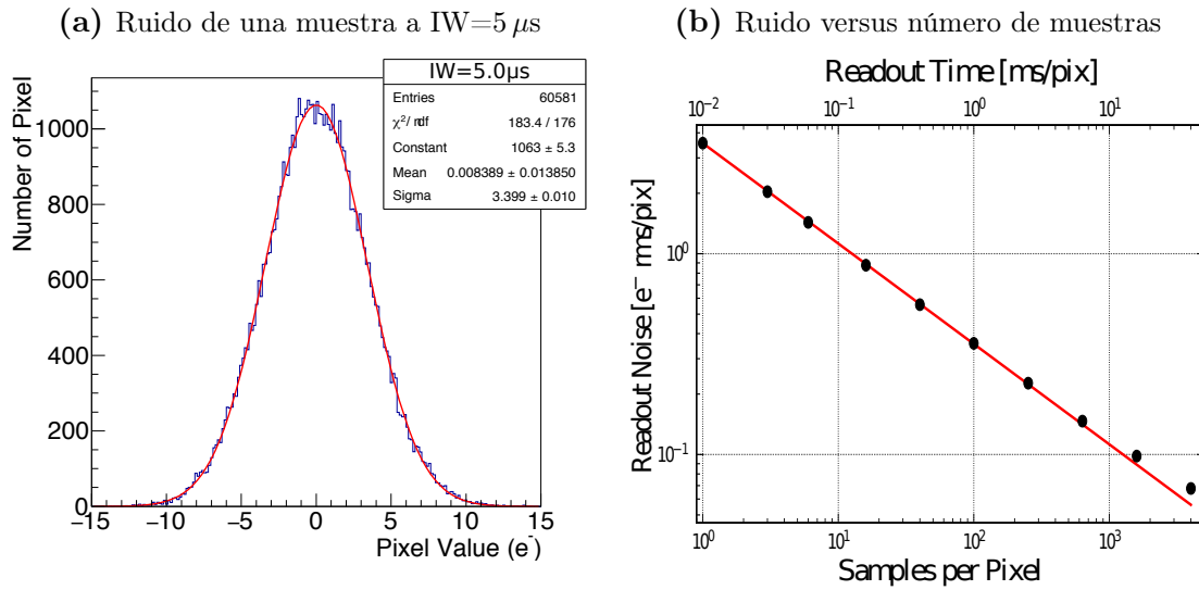
Figura 5.18: En (a) se muestra el ajuste de una función gaussiana con el histograma de píxeles del overscan para un tiempo de integración de 5\mu s . El ruido medido es de 3.399 \pm 0.01 e^- y corresponde al de una única muestra. El ajuste es muy bueno, con \chi^2 = 183,4/176 . En (b) se muestra como decrece el ruido efectivo de lectura con el número de muestras promediadas por pixel. Los puntos negros muestran la desviación estandar de la distribución de píxeles vacíos en función de del número de muestras promediadas. La linea roja es la predicción teórica esperada asumiendo muestras independientes con ruido no correlacionado (ecuación 5.4).
