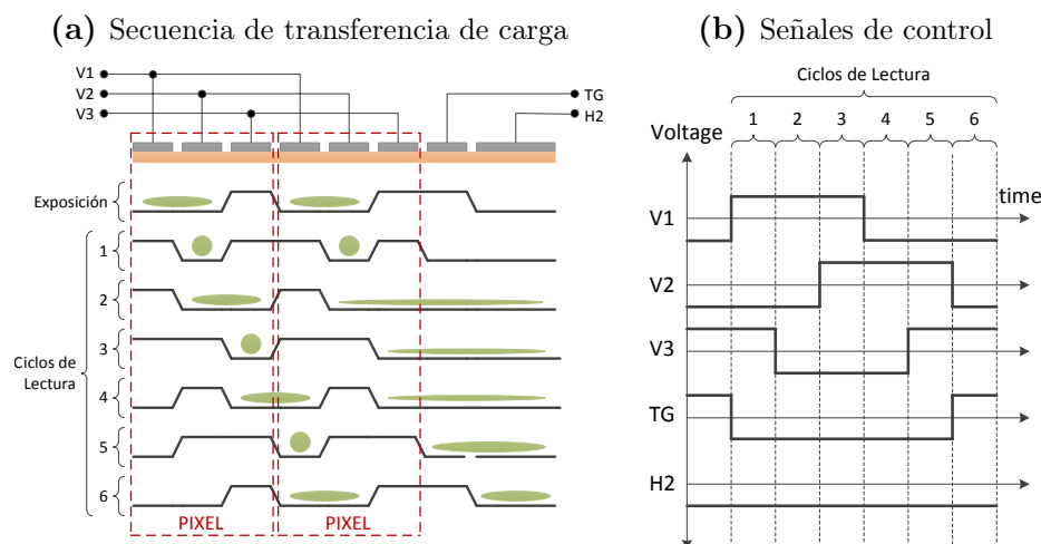
Figura 2.7: En (a) se muestra secuencia de transferencia de carga de los píxeles verticales a horizontal. La burbuja verde representa el paquete de carga del píxel. En (b), se muestra la evolución temporal que deben seguir las señales de control V1, V2, V3 y TG para realizar esa misma secuencia.
