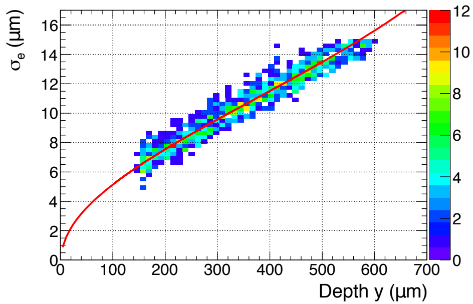
Figura 3.25: Curva tamaño-profundidad para un CCD de 675 \mu\text{m} y 70 V de substrato obtenida utilizando muones. Los puntos fueron obtenidos de 13 muones con dirección perpendicular a las filas de píxeles y de más de 150 píxeles de largo. Solo se utilizan las rebanadas con menos de 1000\text{ e}^- . El ajuste se realizó a partir de y > 150\text{ }\mu\text{m} .
