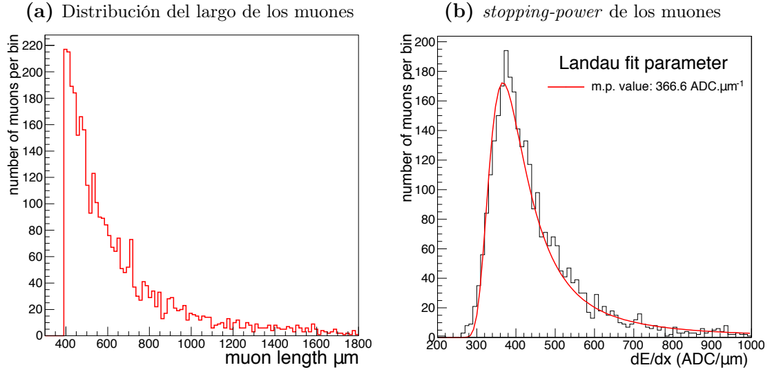
Figura 2.18: Distribución de longitudes de los muones detectados y de stopping-power . Es posible calibrar la ganancia de la cámara con el MPV de la función de Landau.
