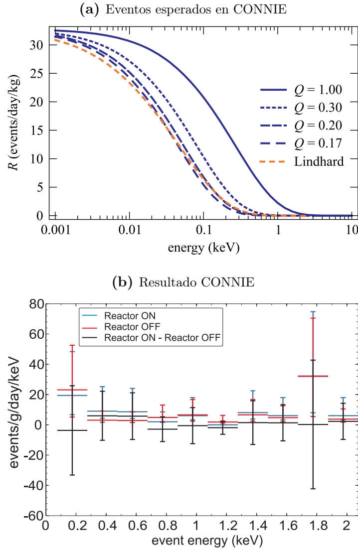
Figura 1.9: En (a) se muestra el número total de eventos esperados con CONNIE en función del umbral de energía mínimo, para diferentes valores de QF (curvas en azul), y usando la teoría de Lindhard (curva naranja). En (b) se muestra el espectro de energía de los eventos detectados con el reactor ON, OFF y su diferencia. Las barras de error son calculadas como la raíz cuadrada del número de eventos de cada bin. El alto rate de eventos en 1.8 keV corresponde al rayo X de fluorescencia del silicio.
