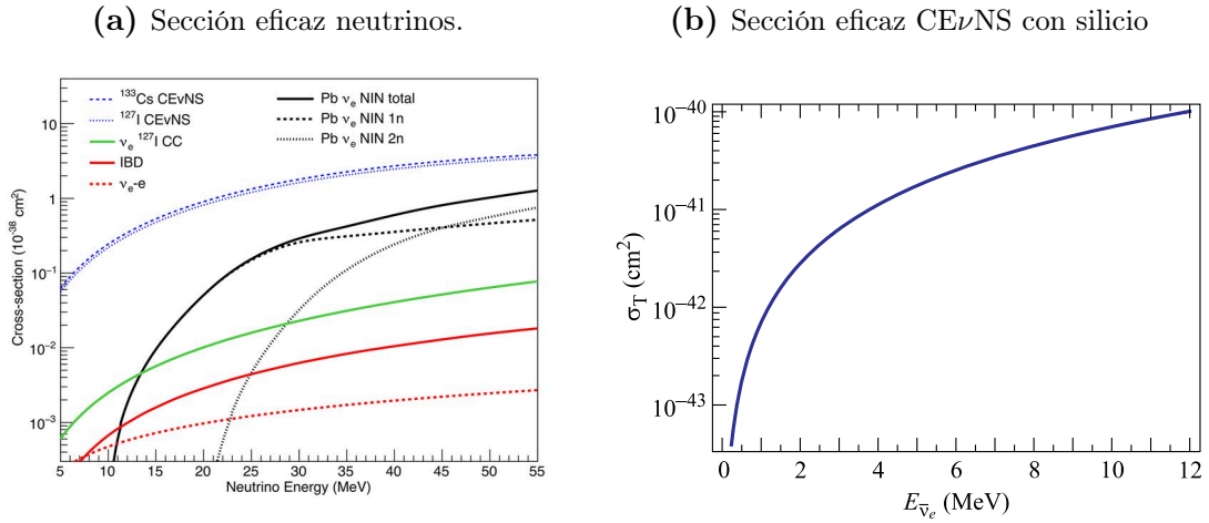
Figura 1.4: En (a) se muestra la sección eficaz total de algunos tipos de interacción (extraída de [5]): dispersión neutrino-electrón, IBD ( inverse beta decay ), NIN (neutrino induced neutron) en plomo, y la más alta es el CE \nu NS con cesio y yodo. En (b) se muestra la sección eficaz total de antineutrinos electrónicos con núcleos de silicio en el rango de energías de neutrinos producidos por un reactor nuclear (extraído de [6]).
