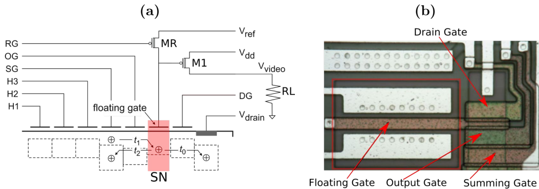
Figura 5.3: En (a) se muestra un diagrama simplificado de la estructura de salida de un skipper CCD. El capacitor MOS con la FG forma el SN (en rojo suave), que permite tomar múltiples muestras del pixel sin destruir la carga. En t_0 la carga en el SN es removida, en t_1 la carga en el SW es transferida al SN, y en t_2 se baja el potencial de OG para volver la carga al SW y comenzar la adquisición de otra muestra. En (b) se muestra una micrografía de la estructura de salida. El transistor dentro del cuadrado rojo es M1.
