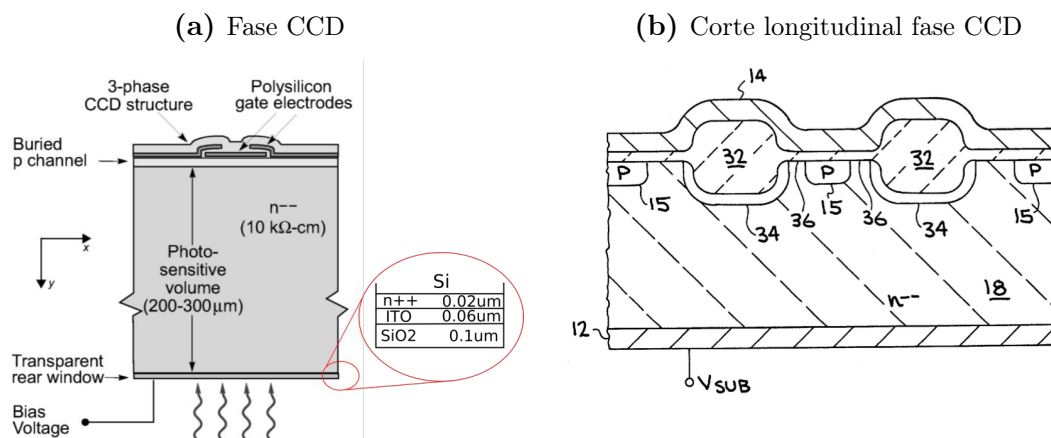
Figura 2.4: En (a) se muestra la sección longitudinal de una fase de un pixel. En el front-side se encuentra el contacto de polisilicio de la compuerta del MOS y en el back-side una serie de capas que reducen la reflexión del infrarrojo. En la figura (b) (extraída de [31]), se muestra un corte transversal de la fase, donde: (34) forma los channel-stops , (15) es el canal de la fase y (32) son regiones de óxido generadas por el proceso de fabricación LOCOS.
