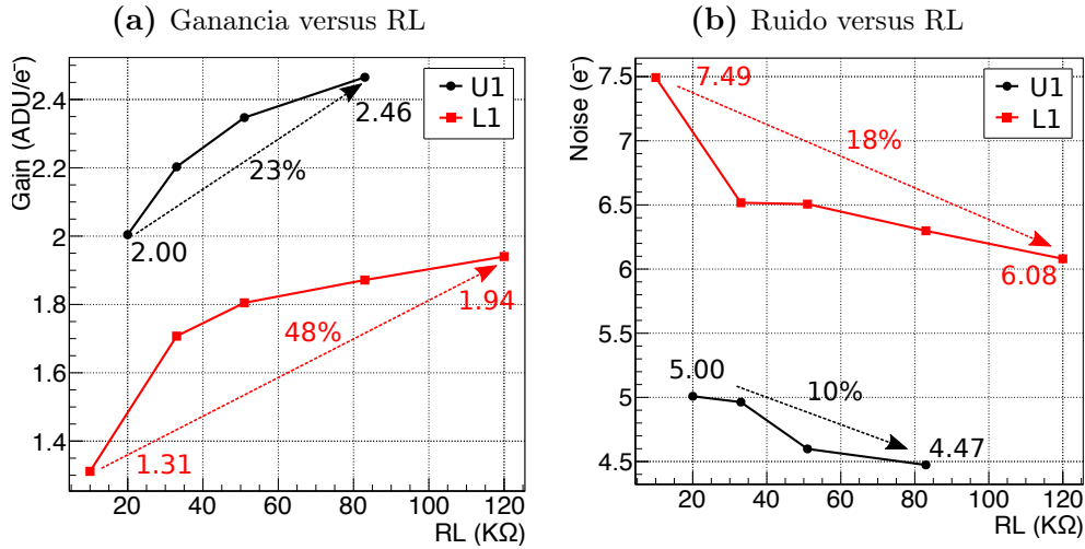
Figura 5.9: Ganancia y ruido a un tiempo de integración de 2.5 \mu s para distintos valores de RL. Como se puede ver, la ganancia aumenta con RL y el ruido en e^- disminuye al mejorar el SNR.
