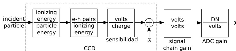
Figura 2.15: Cadena de adquisición de una imagen. La partícula incidente interactúa con el silicio del CCD. Parte de su energía es convertida en pares electrón-hueco. En promedio, a 120 kelvin son necesarios 3.77 eV por par e-h. En el circuito de salida del CCD la carga es convertida a tensión. En la cadena de adquisición es amplificada y procesada por el CDS. Al final, es digitalizada por el ADC.
