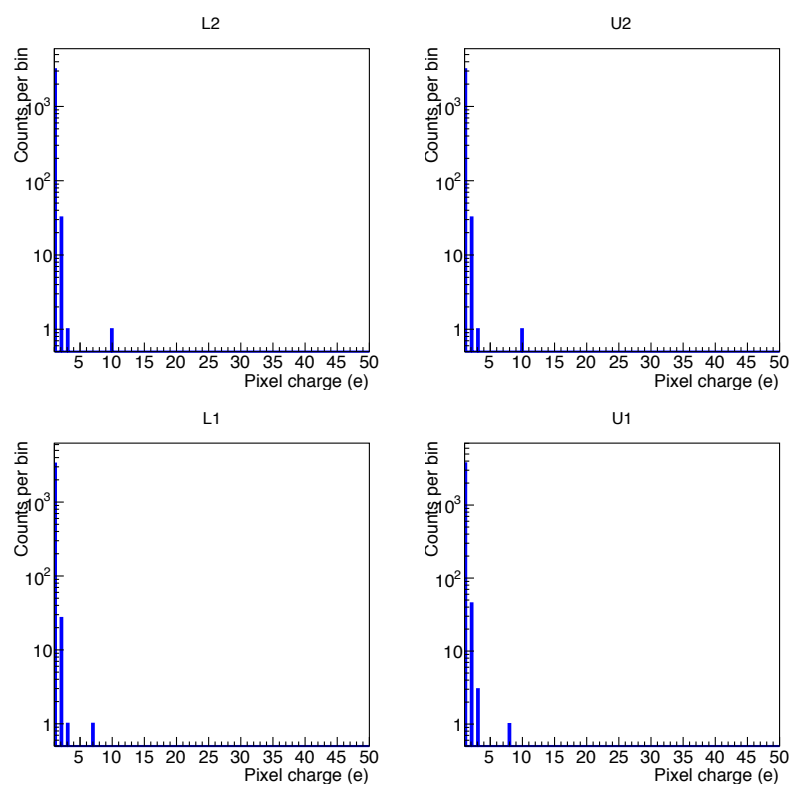
Figura 5.23: Espectro de carga de los eventos detectados por cada cuadrante. Se realizó una adquisición continua de 4 horas de imágenes de 200 líneas (0.032 g). Se detectaron eventos hasta 2 e^- en todos los cuadrantes, compatibles con la frecuencia de carga espuria. Es de destacar que no se detectaron eventos a más de 10 e^- .
