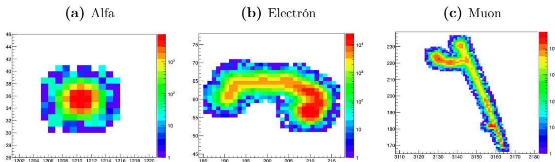
Figura 2.14: Ejemplos de eventos extraídos de las imágenes: (a) fue producido por una partícula alfa y su forma esta definida por el efecto plasma [36]. (b) fue producido por un electrón y el extremo más intenso corresponde al pico de Bragg. En (c) se muestra el evento producido por un muon, en donde se pueden ver dos electrones- \delta .
