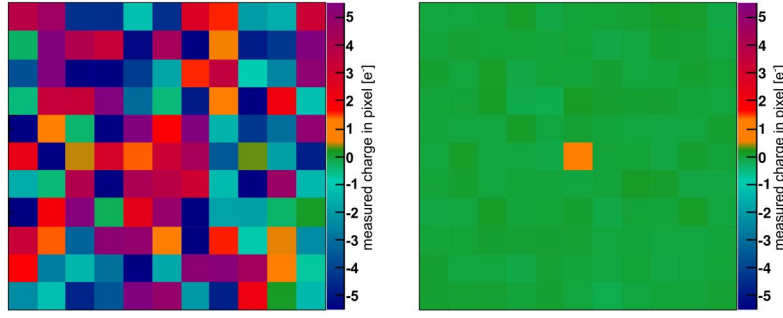
Figura 5.17: A la izquierda se muestra una fracción de imagen con la primera muestra por píxel (un ruido de 4.47 e^- ). Luego de promediar 4000 muestras por píxel el resultado se muestra en la figura derecha. Se puede distinguir que el píxel central tiene un único electrón (color naranja) y los píxeles restantes tienen exactamente cero electrones (color verde).
