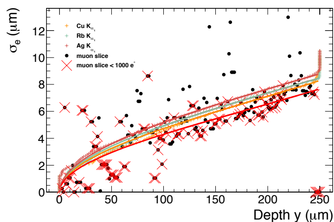
Figura 3.22: En (a) se muestra la distribución de la carga de los segmentos del muon de la figura 3.21a. Se tomaron como segmentos sin electrones- \delta los por debajo de una desviación estándar sobre la media del ajuste gaussiano ( 1000 e^- ). En (b) se muestra la curva tamaño-profundidad obtenida con rayos X y utilizando el muon de la figura 4.5. Los puntos negros corresponden a cada rebanada de un pixel del muon, y los marcados con una cruz roja son aquellas con menos de 1000 e^- .
