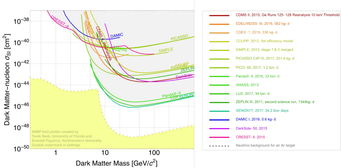
Figura 1.6: Espacio de parámetros de WIMP explorado por diferentes experimentos, los límites de exclusión tienen un nivel de confianza del 90 %. Por debajo de 10 \text{ GeV}/c^2 el espacio de parámetros se encuentra muy poco explorado.
