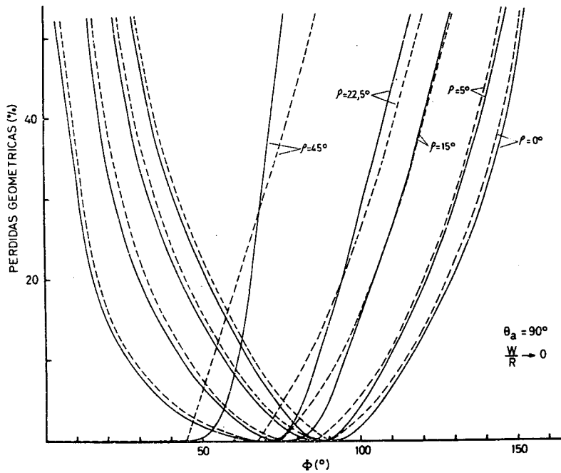
Fig. 5: Pérdidas geométricas en un CFEF, en función de \phi , para las dos disposiciones de los espejos consideradas y varios valores de \rho . Criterio 1: ---- ; criterio 2: — .
