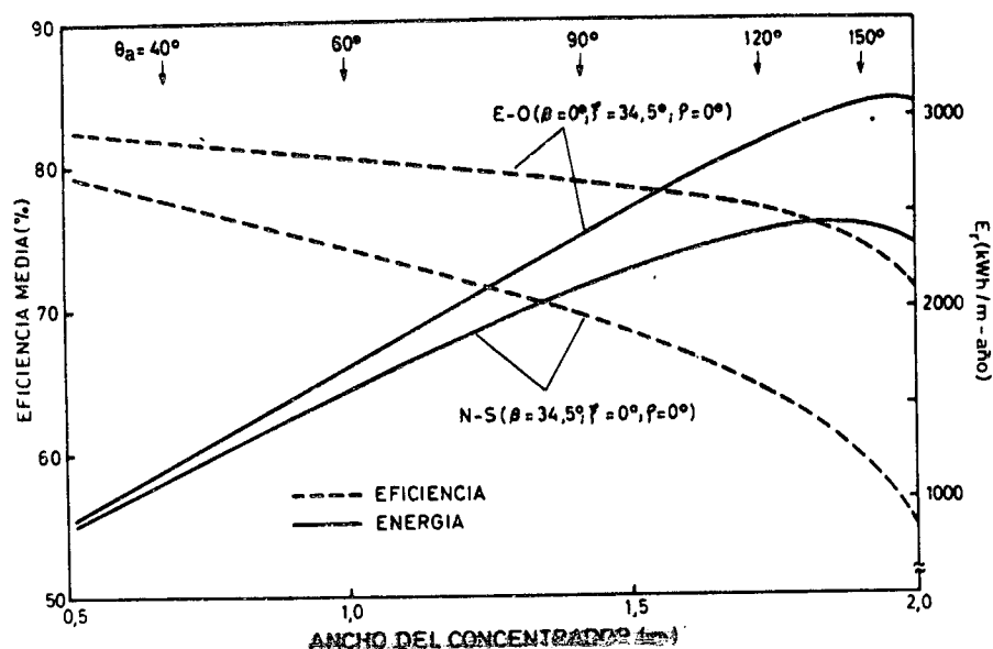
Fig. 8: Eficiencia media anual y energía incidente en el receptor a lo largo de un año (por unidad de longitud del concentrador) en función del ancho de un CFEF con R = 1 m, ubicado en Buenos Aires con orientación E-0 o N-S.
