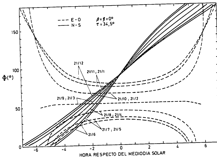
Fig. 2: Variación diaria de \phi para distintas épocas del año, considerando un concentrador con \xi = \beta = 0 ubicado a 34^{\circ}30'S .
