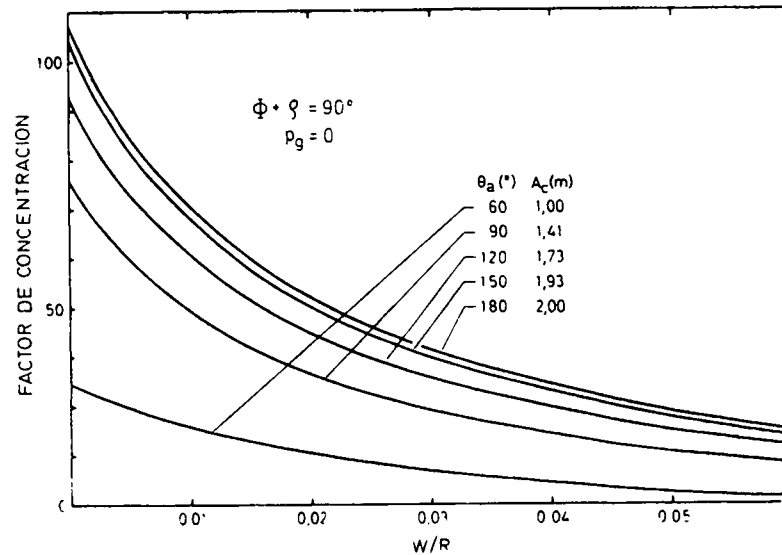
Fig. 6: Factor de concentración de un CFEF en el cual se cumple la condición \phi + \gamma = 90^\circ (ver Fig. 5) y, por lo tanto, p = 0 , en función de W/R , para distintos valores del ángulo de apertura \theta_a (y del correspondiente ancho A_c del concentrador si R = 1 m.)
