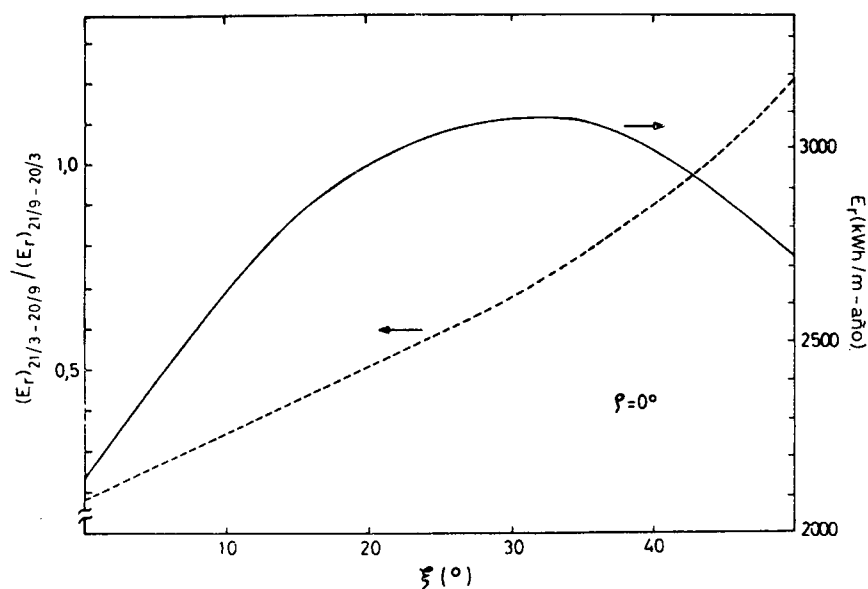
Fig. 9: Energía incidente en el receptor a lo largo de un año y relación y entre las que inciden en los períodos 21/3-20/9 y 21/9-20/3, en función del ángulo. Se ha realizado el cálculo para un concentrador con orientación E-0, ubicado en Buenos Aires, con un ángulo de abertura de 150^\circ y con un radio de 1 m. La energía anual incidente está dada por unidad de longitud del concentrador.
