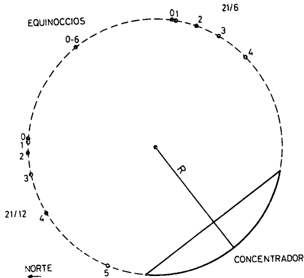
Fig. 3: Variación diaria de la posición del foco lineal en un CFEF ubicado a 34^{\circ}30'S con orientación E-0 y con \beta = 0 y \xi = 34^{\circ}30' . Los números identifican horas antes o después del mediodía solar, correspondientes a cuatro épocas del año.
