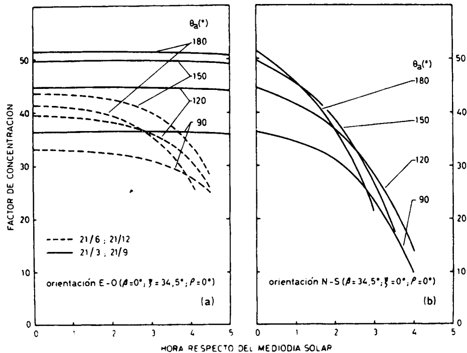
Fig. 7: Variación diaria del factor de concentración de un CFEF con W/R = 0,02 ubicado a 34,5^\circ S para distintos ángulos de apertura \theta_a . (a) Orientación E-O. Factores de concentración máximo y mínimo logrables en el año. (b) Orientación N-S. El factor de concentración es constante a lo largo del año.
