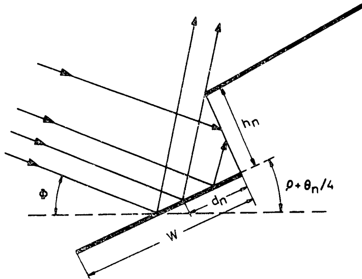
Fig. 4: Proyección de dos espejos sucesivos sobre un plano perpendicular al eje de simetría del cilindro directriz, para un concentrador con \xi = 0 . W es el ancho del espejo; h_n la distancia entre los bordes de los espejos n y n+1 y d_n la parte del espejo n caracterizada porque la luz reflejada desde ella es interceptada antes de llegar al receptor. Según Ref. 3.
