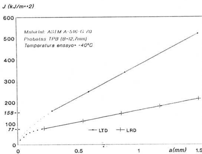
Fig. 3. Curvas J-R
