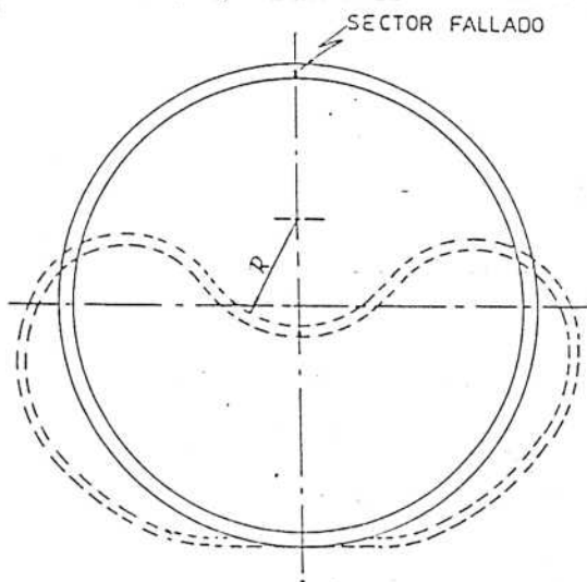
Fig. 1. Detalle de deformaciones postuladas
