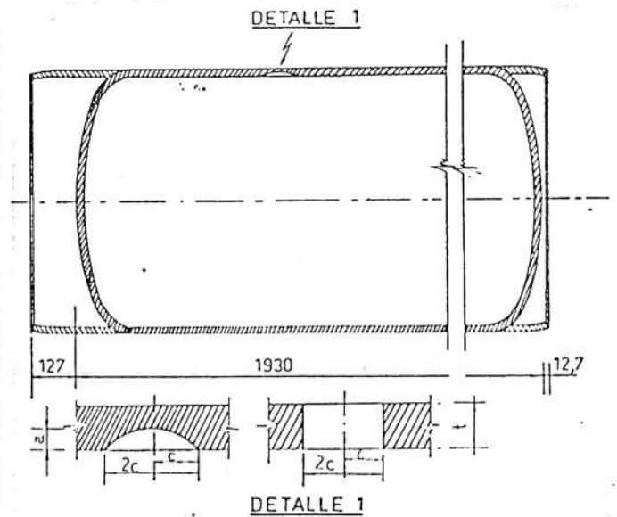
Fig.2. Descripción del componente
