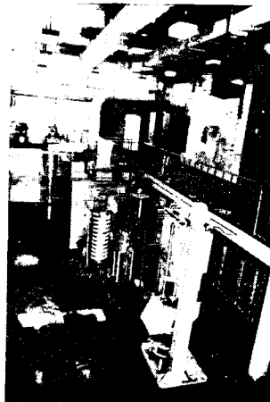
F. 27 Planta de tratamiento de residuos sólidos de baja actividad (Centro Atómico Ezeiza).
