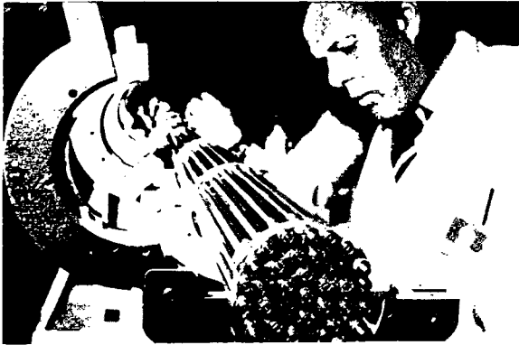
F. 20 Armado de un prototipo de elemento combustible Atucha (Centro Atómico Constituyentes).
