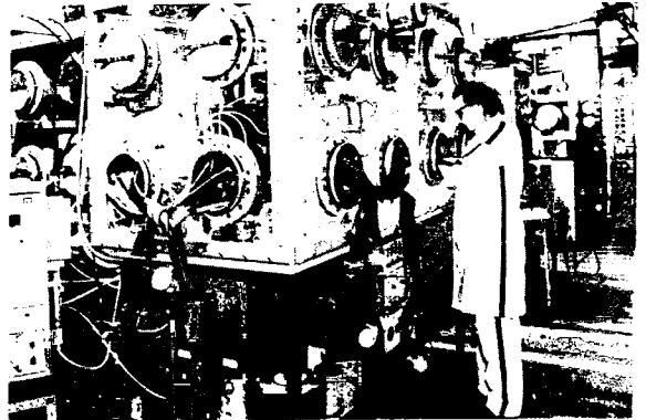
F. 22 Laboratorio para trabajo con materiales alfa-activos (Centro Atómico Constituyentes).
