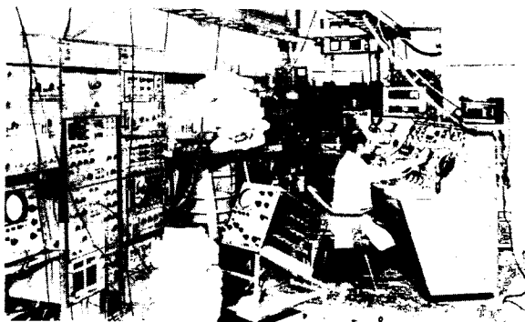
F. 30 Instalación para estudios de esquemas de desintegración de radio-nucleídos de vida media muy corta (Sede Central).
