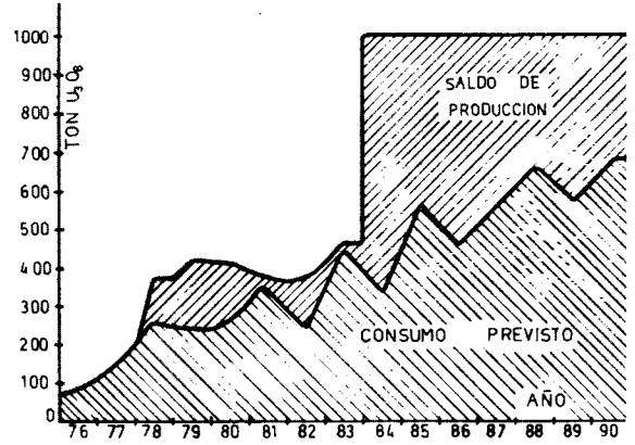
F. 16 Evolución prevista para la producción de concentrado de uranio.
