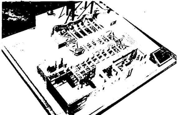
F. 26 Maqueta de la planta de irradiación gamma (Centro Atómico Ezeiza).
