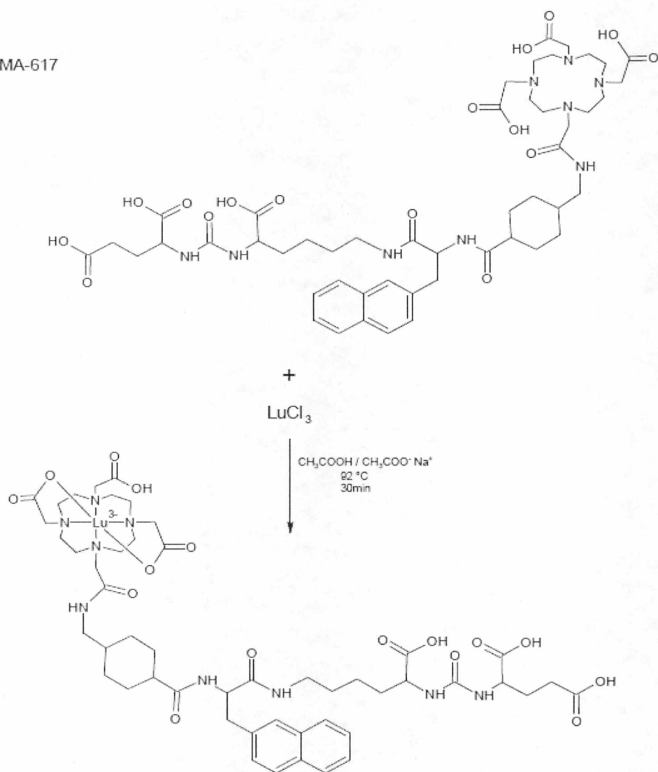
Figura 6: esquema de radiosíntesis del ^{177}\text{Lu} -PSMA-617.
