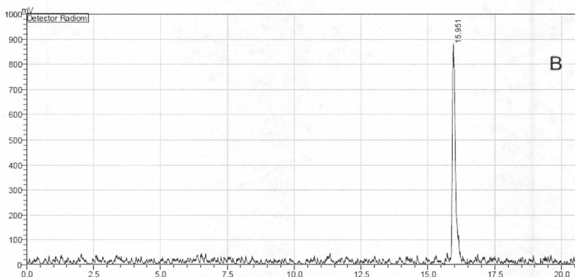
Figura 14: Radio cromatogramas de HPLC en fase reversa para ^{177}\text{Lu} -PSMA-617, Marcación 5. Gráficos A: luego de la marcación, B: a las 24 horas.
