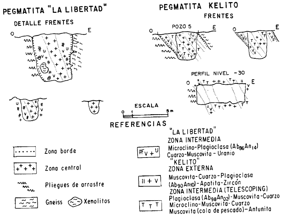
Fig. 6. — Corte transversal de las pegmatitas « La Libertad » y « Kelito »
