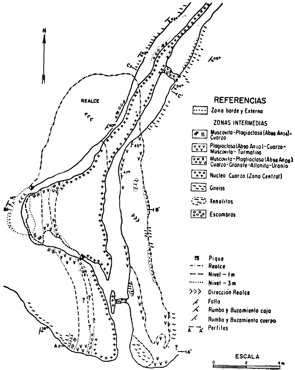
Fig. 7. — Estructura zonal en la pegmatita «Elsa»
