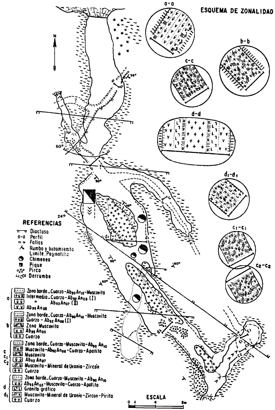
Fig. 5. — Estructura zonal en la pegmatita « El Desmorre ».
