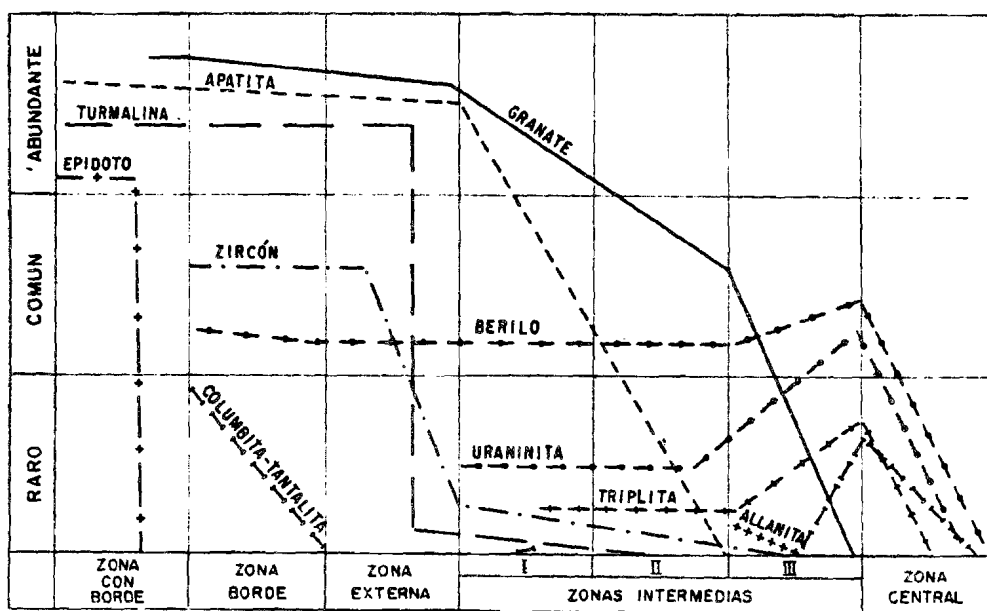
Fig. 10. — Distribución de los minerales accesorios según su abundancia
