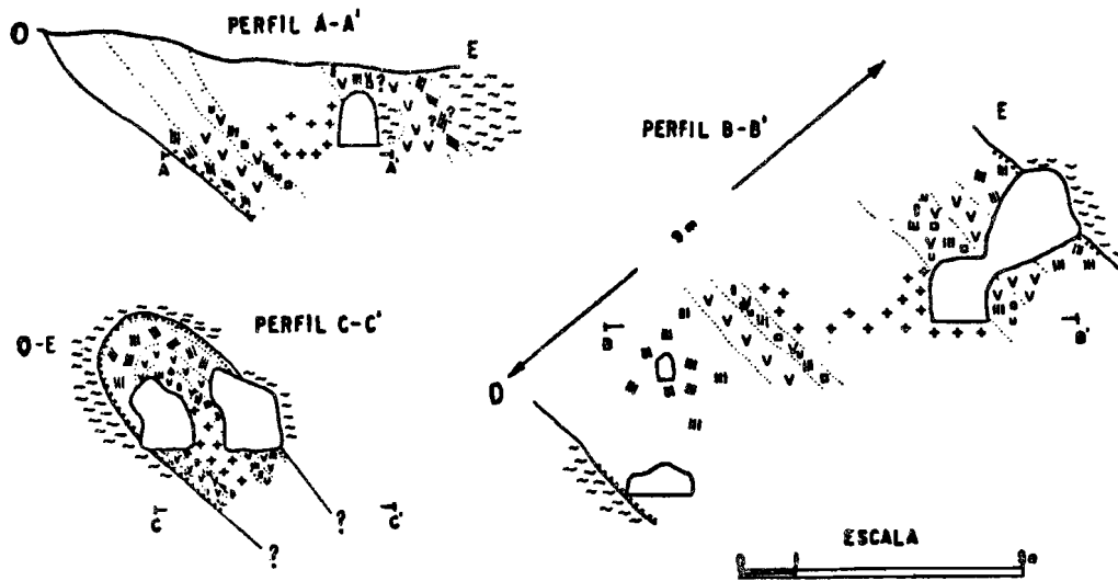
Fig. 2. — Perfil en la pegmatita C° Blanco (« Los Guardias »)
