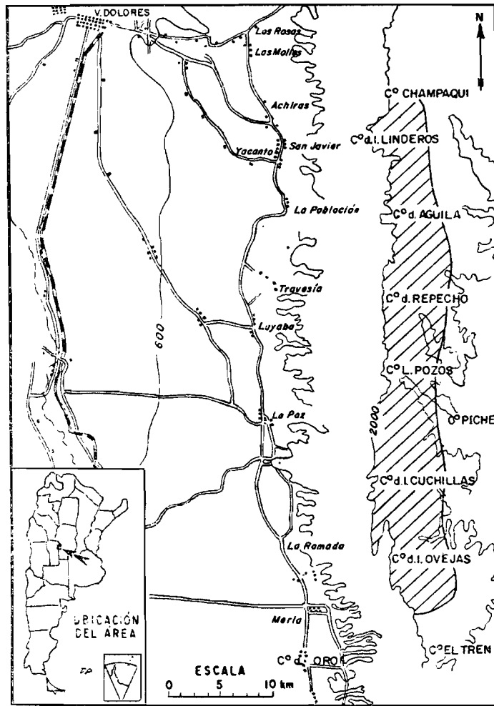
Fig. 1. — Croquis de ubicación. ///, área de observaciones
