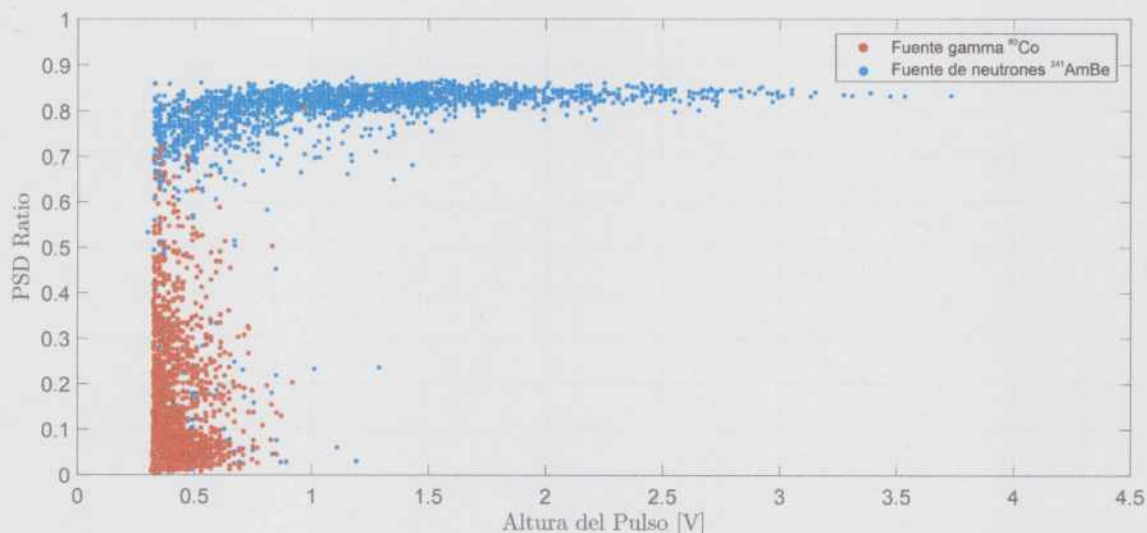
Figura 4.10: Análisis del cociente PSD en función de la altura de los pulsos para el detector #09 (inorgánico con 6 Li al 90 %). Se observa la separación de las dos poblaciones atribuidas a neutrones y fotones gamma.
