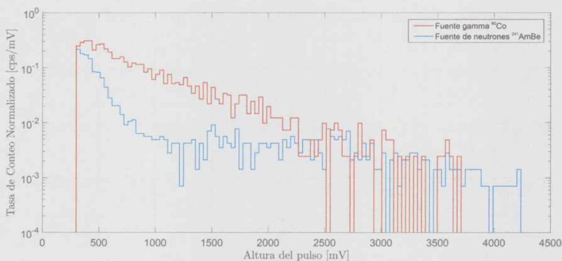
Figura 4.5: Espectros diferenciales de altura de pulsos normalizado obtenidos con el detector #25 (orgánico con ^6\text{Li} al 90 %).
