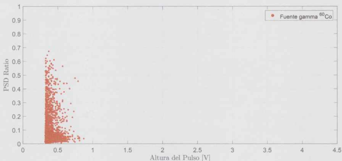
Figura 4.16: Análisis del cociente PSD en función de la altura de los pulsos para el detector #09 (inorgánico con {}^6\text{Li} al 90 %) con la fuente de {}^{60}\text{Co} .
