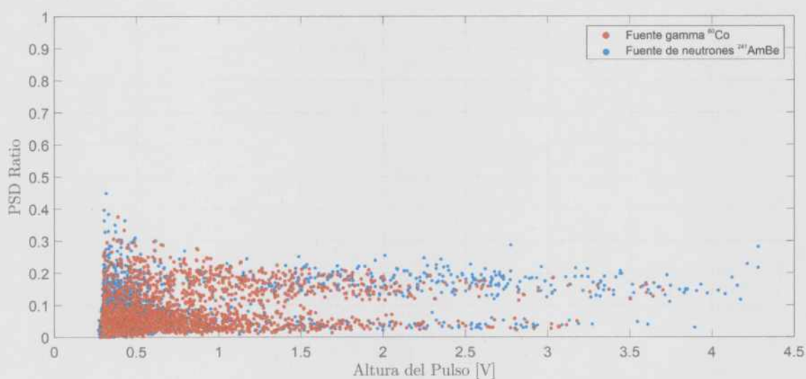
Figura 4.8: Análisis del cociente PSD en función de la altura de los pulsos para el detector #25 (orgánico con ^6\text{Li} al 90 %). Se observa que las poblaciones de neutrones y fotones gamma se solapan.
