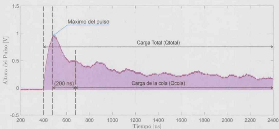
Figura 4.3: Elección del comienzo de la cola del pulso para el cálculo del cociente PSD.
