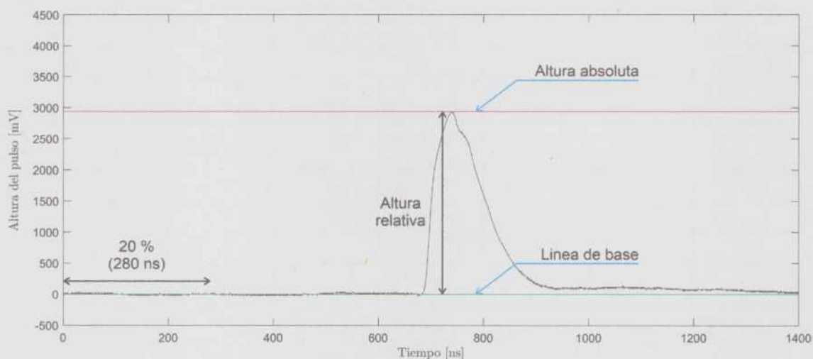
Figura 4.2: Análisis de la altura relativa de un pulso típico.
