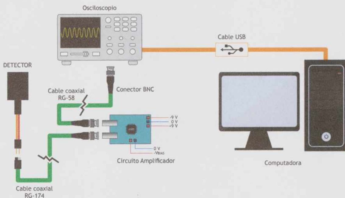
Figura 4.1: Esquema de la configuración 2 utilizada en los experimentos mencionados en este Capítulo.
