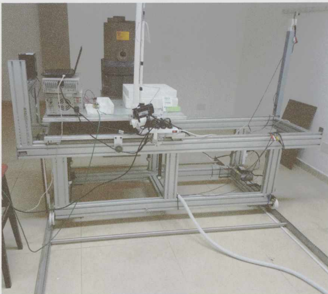
Figura 4.12: Banco motorizado utilizado para desplazar el dispositivo a irradiar a distintas distancias de la fuente.
