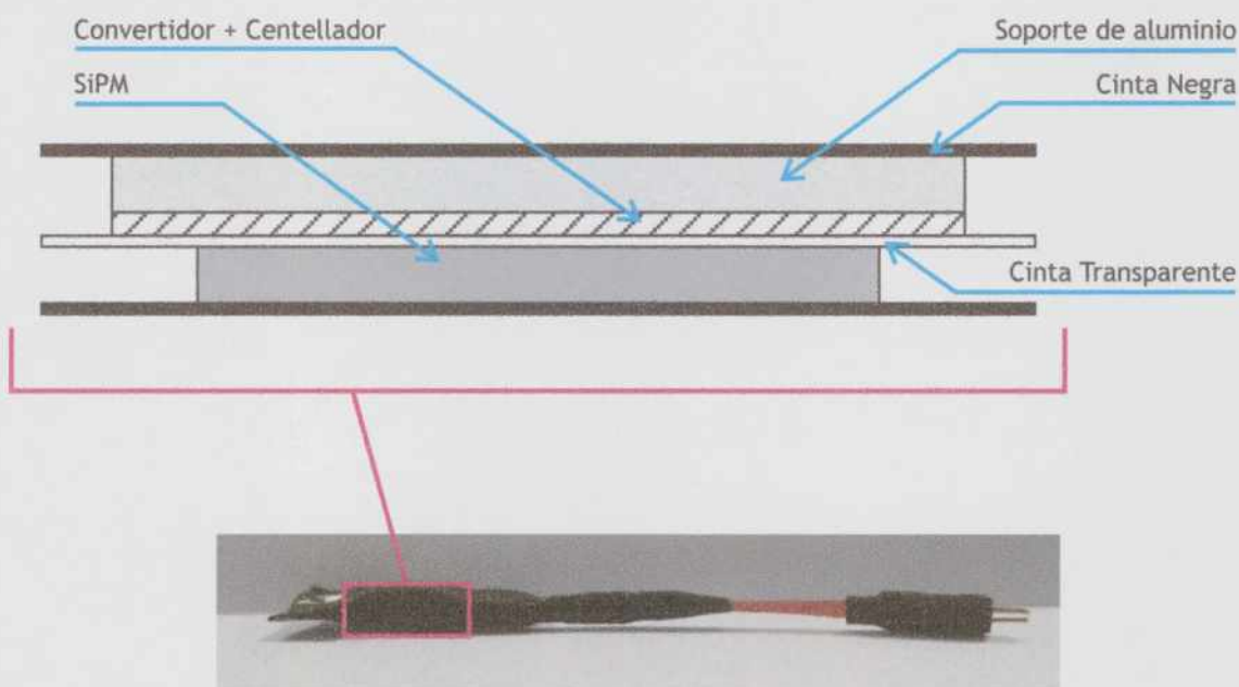
Figura 3.1: Esquema del ensamble fotodetector-centellador.
