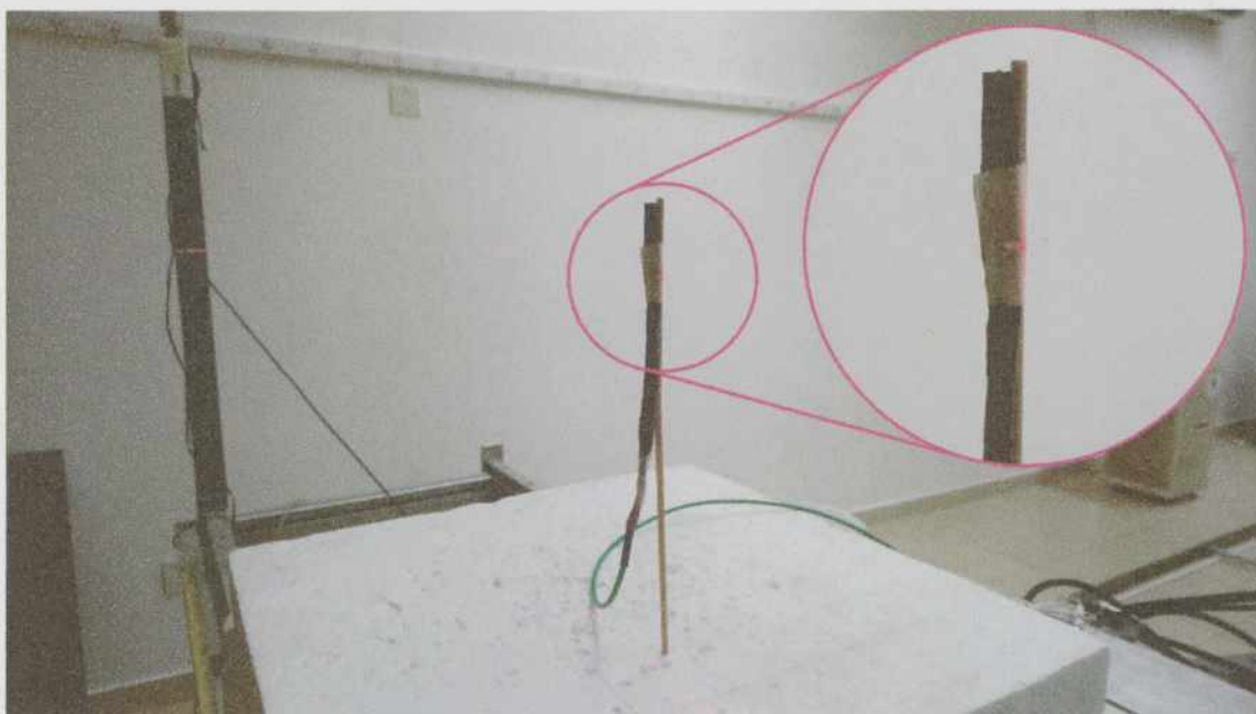
Figura 4.13: Detector colocado en la posición de irradiación. En la imagen se observa uno de los láseres marcando con precisión el lateral del detector.
