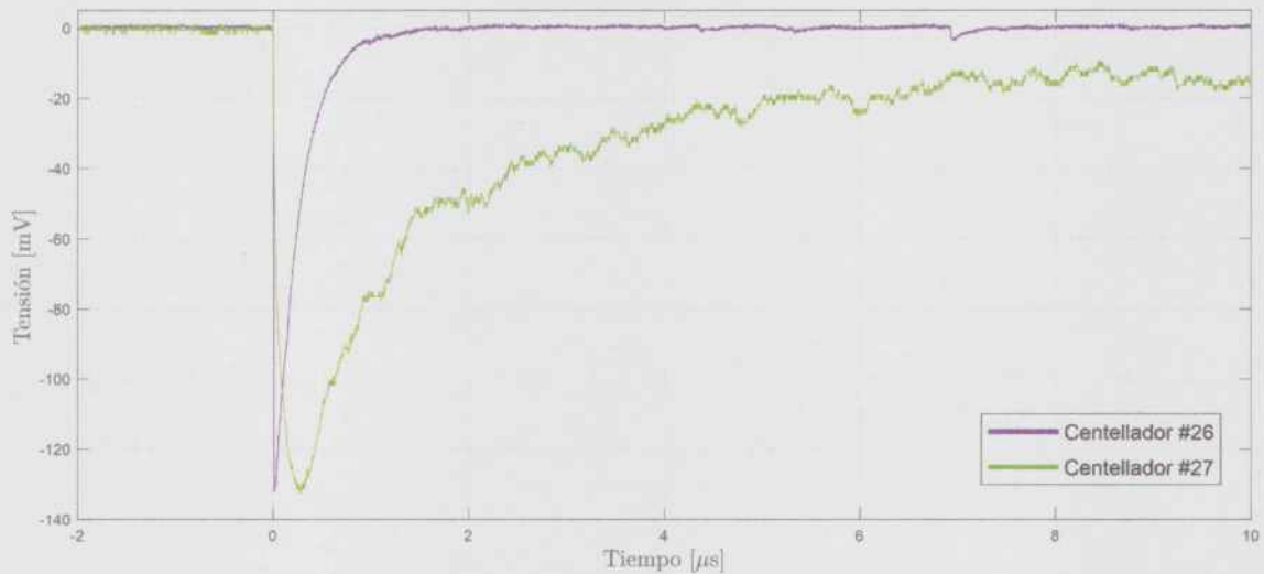
Figura 3.7: Pulsos característicos de los centelladores orgánicos (representado por el compuesto #26) e inorgánicos (representado por el compuesto #27) ensayados en este Trabajo.
