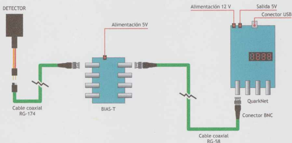
Figura 3.2: Esquema de la configuración 1 utilizada en los experimentos mencionados en este Capítulo.
