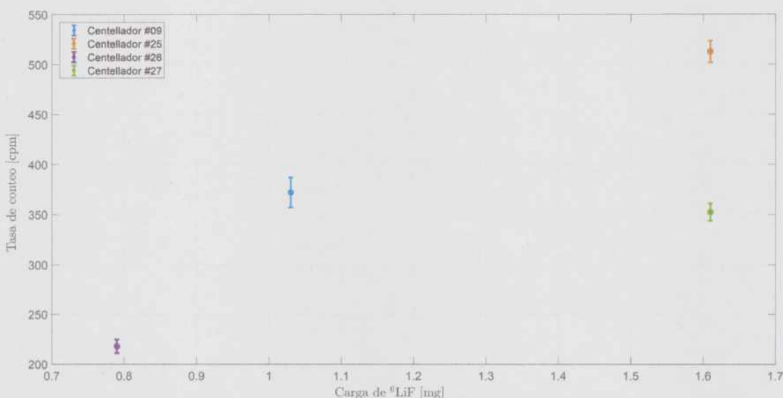
Figura 3.5: Variación de la tasa de conteo de los detectores ensayados en función de la carga de ^6\text{LiF} . Se muestran los resultados de los centelladores #09 (inorgánico con ^6\text{Li} al 90 %, preparado con aerógrafo), #25 (orgánico con ^6\text{Li} al 90 %, preparado con pipeta), #26 (orgánico con Li natural, preparado con pipeta) y #27 (inorgánico con ^6\text{Li} al 90 %, preparado con pipeta).
