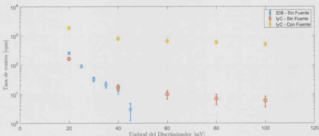
Figura 3.4: Variación de la tasa de conteo en función del umbral del discriminador para tres mediciones con el detector #9.
