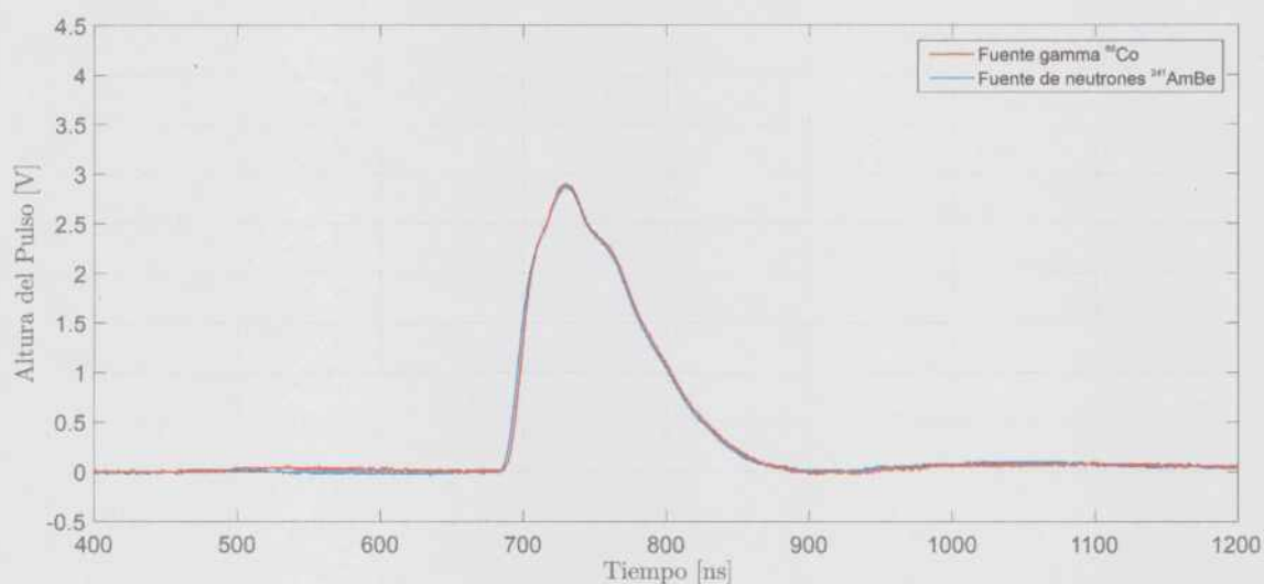
Figura 4.7: Pulsos típicos obtenidos con el detector #25 (orgánico con ^6\text{Li} al 90 %) utilizando la fuente de neutrones y la fuente de fotones gamma.
