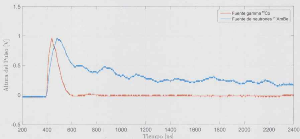
Figura 4.9: Pulsos típicos obtenidos con el detector #09 (inorgánico con 6 Li al 90 %) utilizando la fuente de neutrones y la fuente de fotones gamma.
