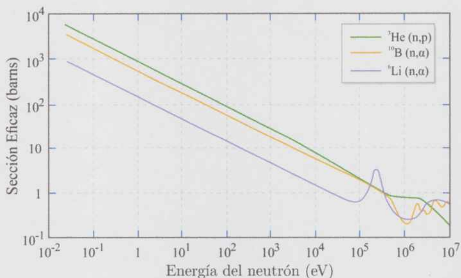
Figura 2.2: Sección Eficaz Total en función de la energía del neutrón incidente para los nucleidos más utilizados en detección de neutrones térmicos.
