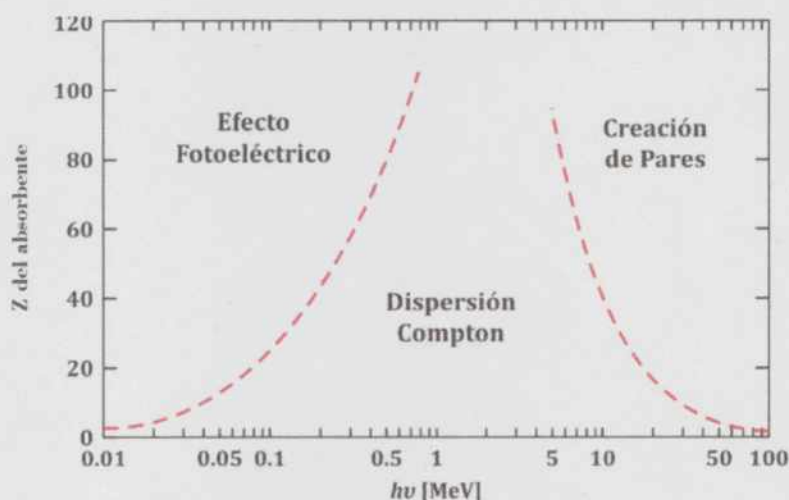
Figura 2.1: Mecanismos de interacción más probables en función de la energía del fotón y el Z del material absorbente.
