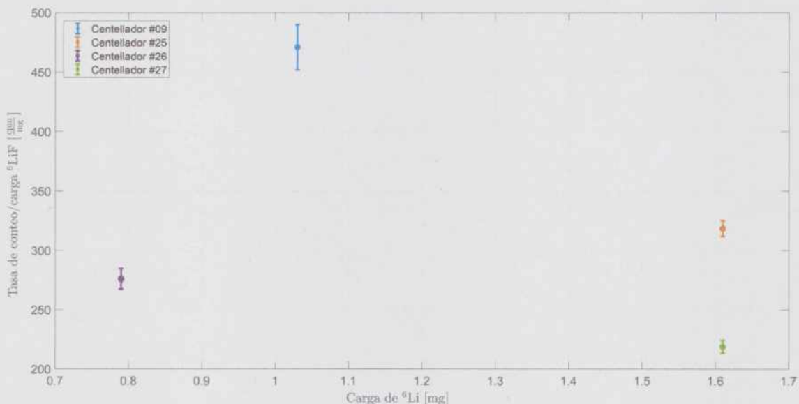
Figura 3.6: Aprovechamiento de la carga de ^6\text{LiF} en términos de la tasa de conteo obtenida por el detector. Se muestran los resultados de los centelladores #09 (inorgánico con ^6\text{Li} al 90 %, preparado con aerógrafo), #25 (orgánico con ^6\text{Li} al 90 %, preparado con pipeta), #26 (orgánico con Li natural, preparado con pipeta) y #27 (inorgánico con ^6\text{Li} al 90 %, preparado con pipeta).
