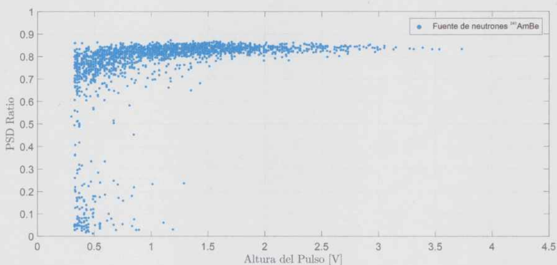
Figura 4.17: Análisis del cociente PSD en función de la altura de los pulsos para el detector #09 (inorgánico con ^6\text{Li} al 90 %) con la fuente de ^{241}\text{AmBe} .
