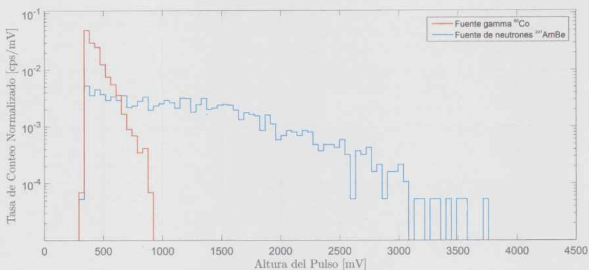
Figura 4.6: Espectros diferenciales de altura de pulsos normalizado obtenidos con el detector #09 (inorgánico con ^6\text{Li} al 90 %).
