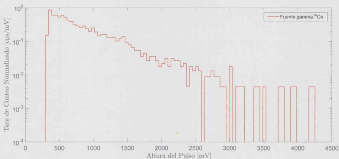
Figura 4.14: Espectro diferencial de altura de pulsos de la fuente de ^{60}\text{Co} obtenido con el detector #25 (orgánico con ^6\text{Li} al 90 %).
