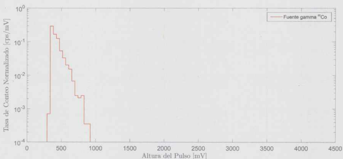
Figura 4.15: Espectro diferencial de altura de pulsos de la fuente de ^{60}\text{Co} obtenido con el detector #25 (orgánico con ^6\text{Li} al 90 %).
