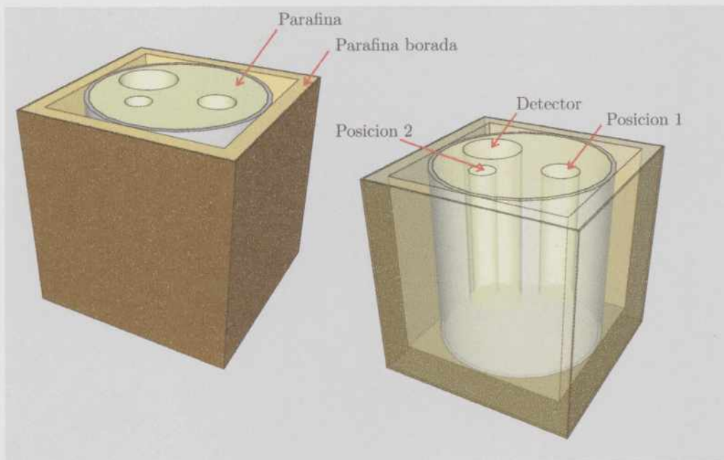
Figura 3.3: Esquema del bloque moderador y blindaje utilizado en los experimentos mencionados en este Capítulo.
