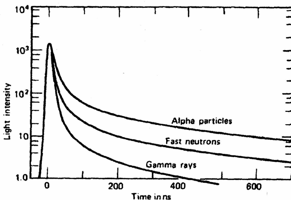
Figura 2.3: Dependencia del tiempo de decaimiento del pulso con la partícula incidente para un centellador orgánico.
