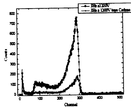
Espectro de altura de pulsos de un detector proporcional de 3He
