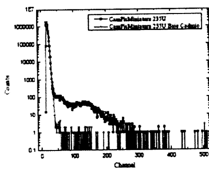
Espectro de altura de pulsos de una cámara de ionización. Cámara de fisión miniatura de 235U
