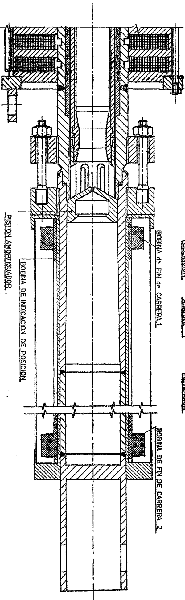
MECANISMO DE ACCIONAMIENTO Y DE INDICACION DE POSICION DE LAS BARRAS DE CONTROL
