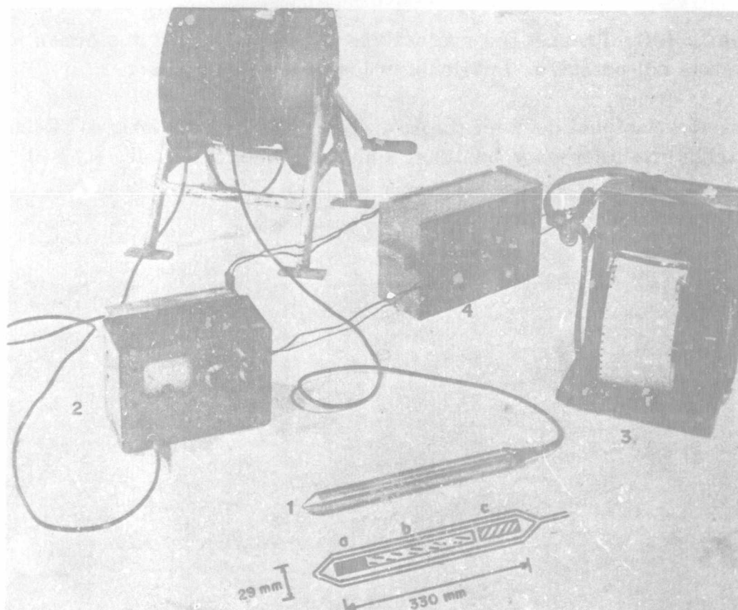
Fig. 2. Instrumental electrónico empleado en las mediciones de actividad 1.a) Sonda detectora con cristal de Ina(Tl) b) Fotomultiplicador c) Preamplificador 2. ) Integrador transistorizado 3. ) Registrador gráfico mecánico 4. ) Fuente de tensión
